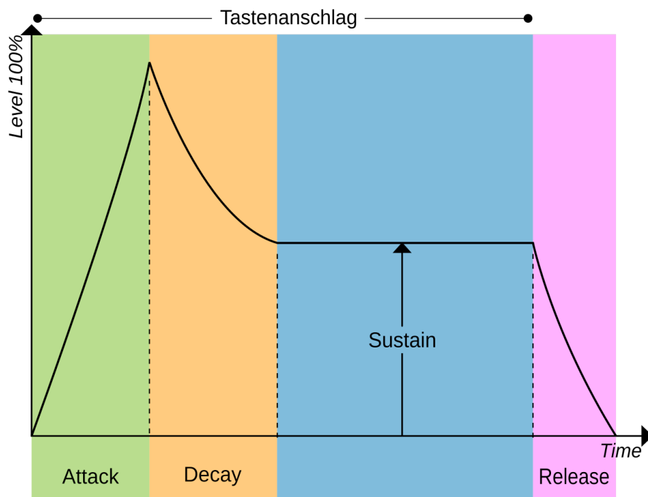
Rysunek 2.1: Schematyczna wizualizacja obwiedni dźwięku ADSR (oś pionowa: amplituda, oś pozioma: czas) [25].
