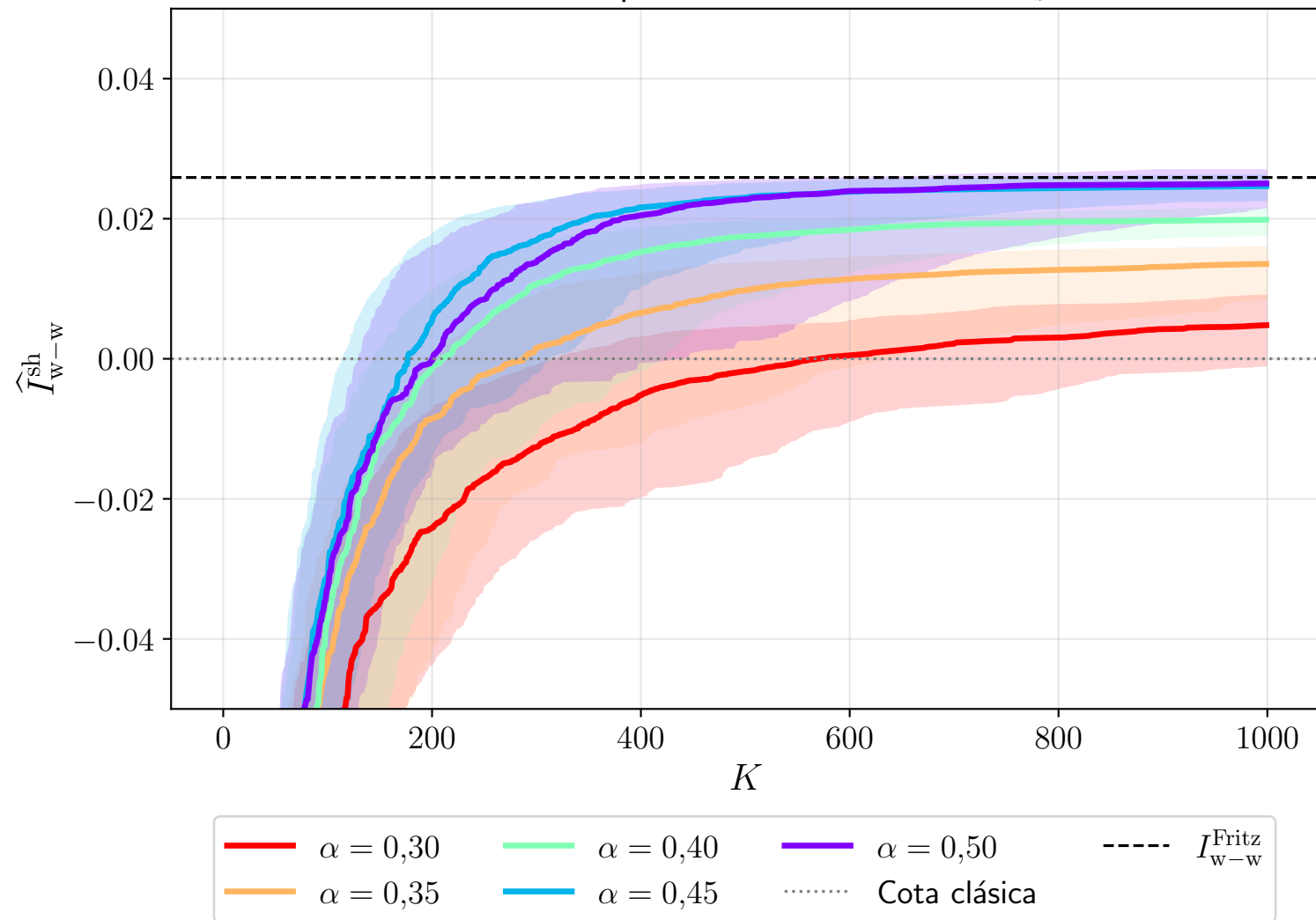
Estados en descomposición de Schmidt con N_{\text{sh}} = 10^6
