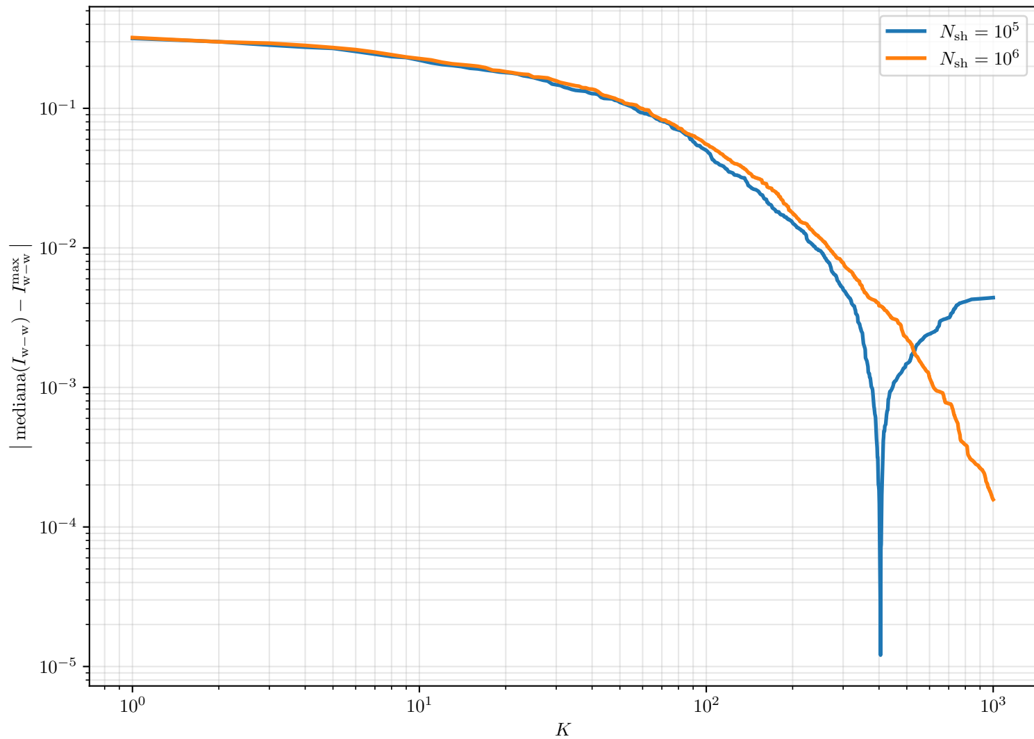
Sim01_02 — Distancia al máximo cuántico, N_{\text{sh}} = 10^5 vs 10^6
