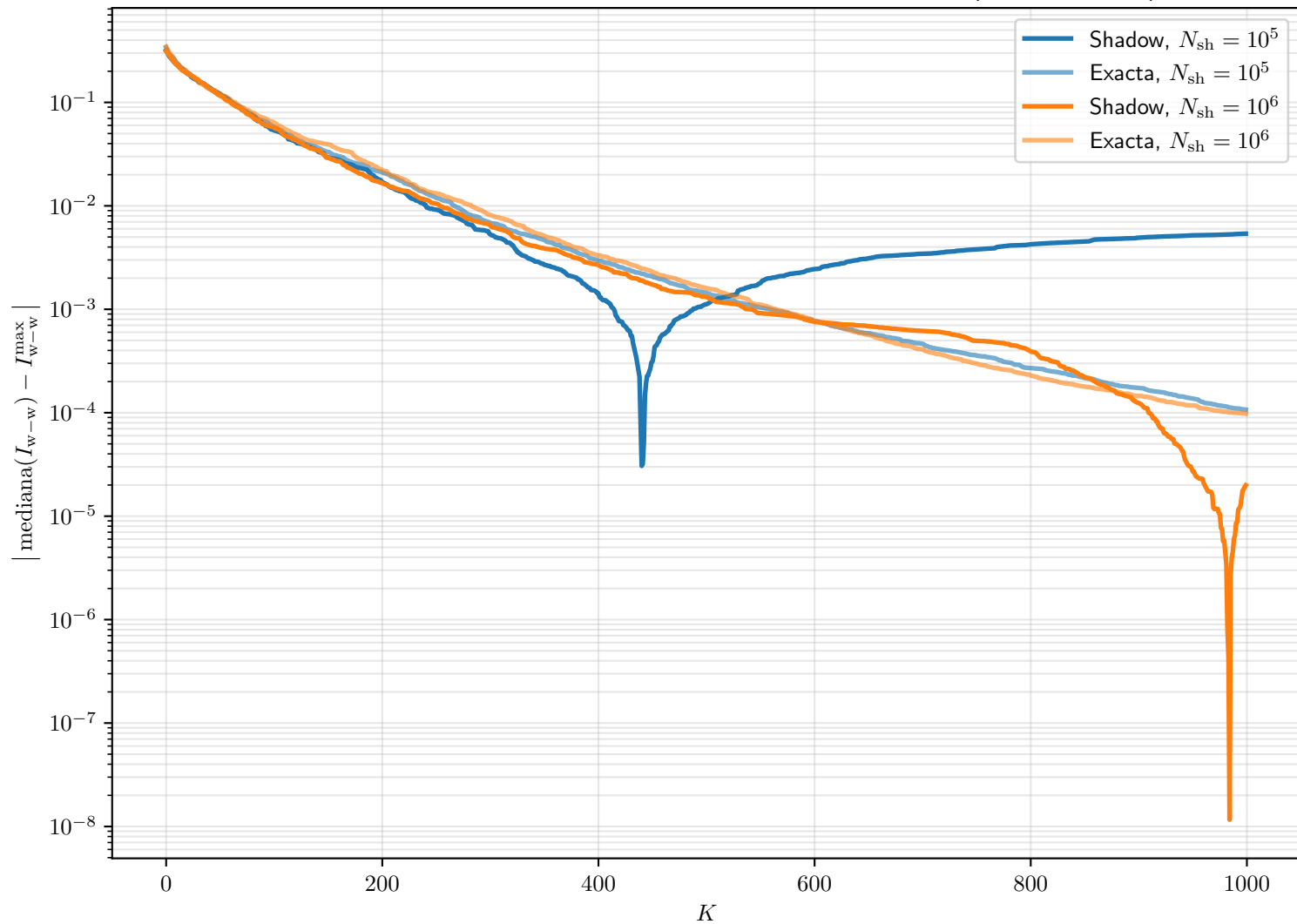
Sim01_03 — Distancia al máximo cuántico, Exacta vs Shadow ( N_{\text{sh}} = 10^5, 10^6 )
