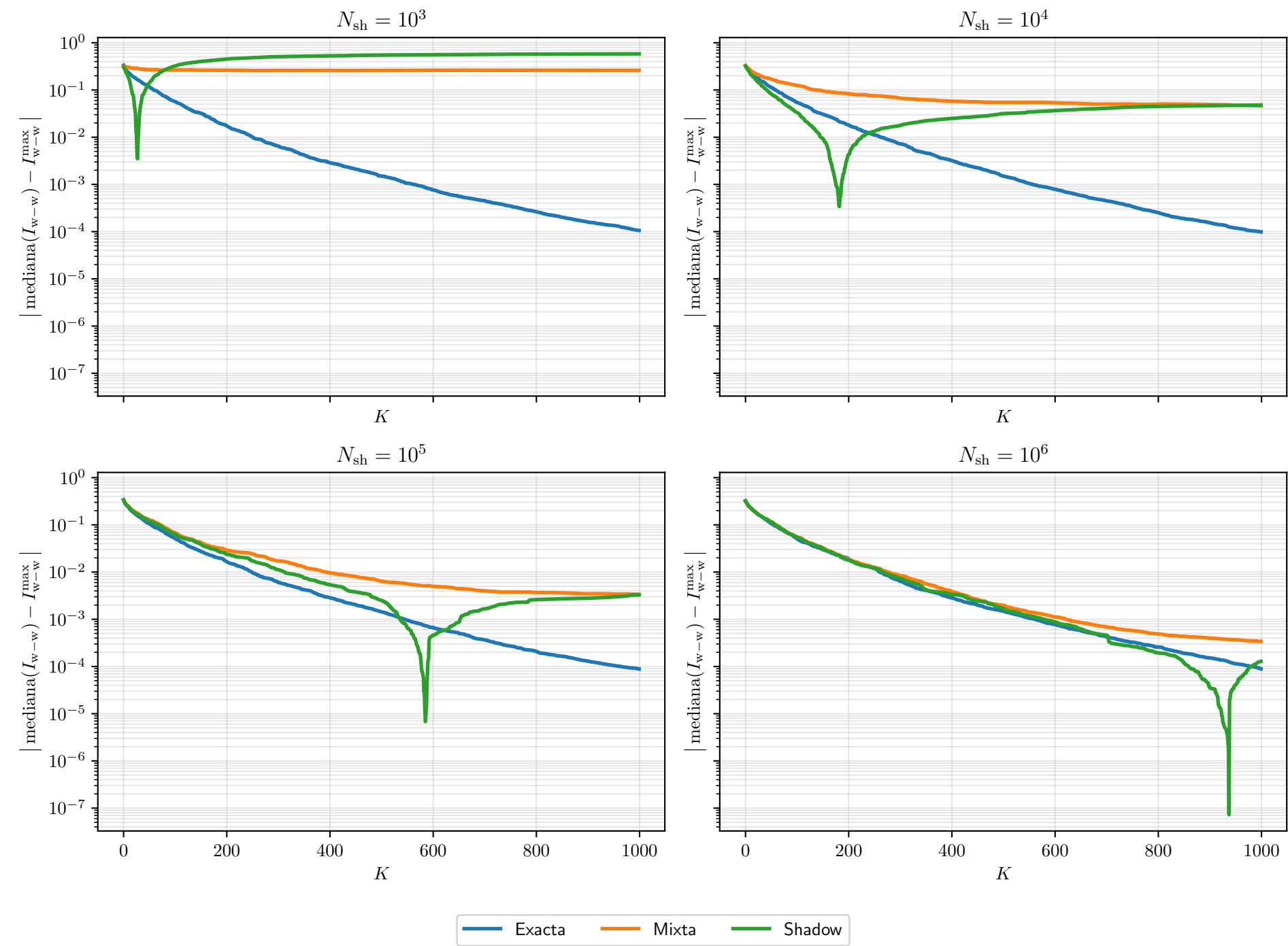
Sim01_04 — Distancia al máximo cuántico, Exacta vs Mixta vs Shadow por N_{\text{sh}}
