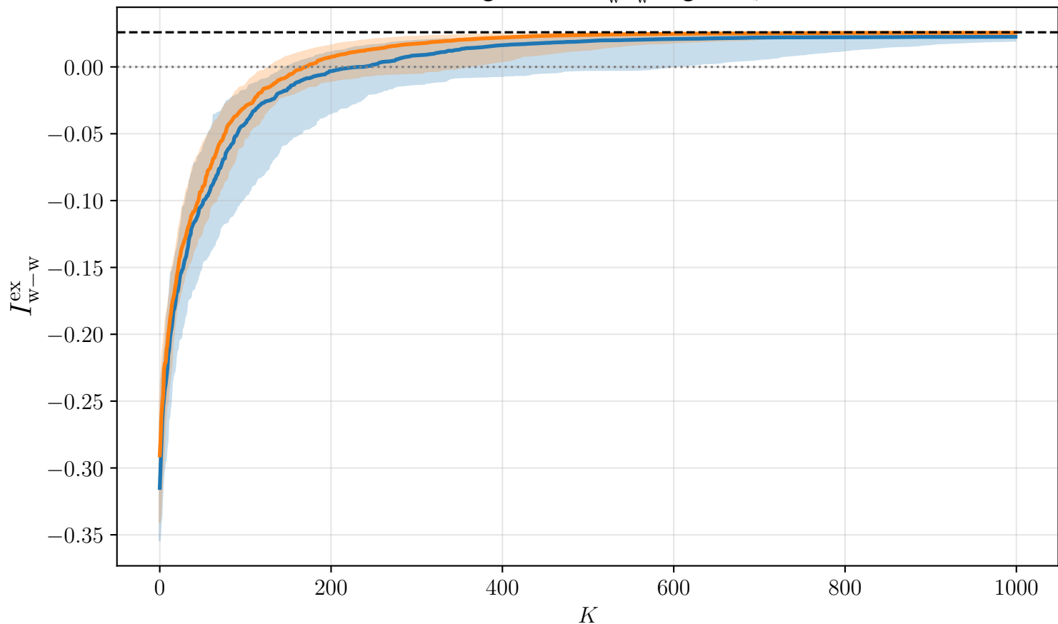
Convergencia de I_{w-w}^{\text{ex}} según N_{\text{sh}}
