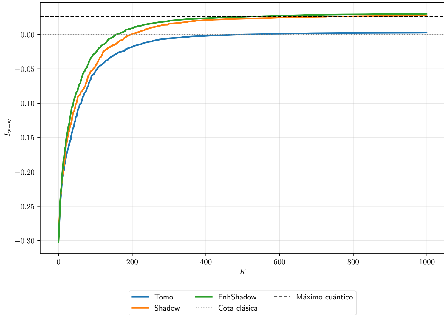
Simulación 01 — Mediana de convergencia, estado maximalmente entrelazado
