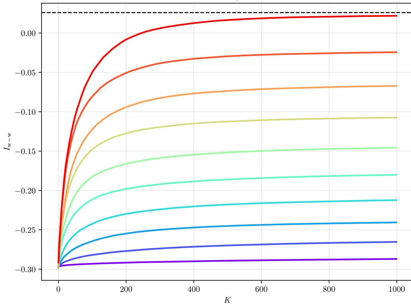
Mediana de convergencia de I_{w-w}
