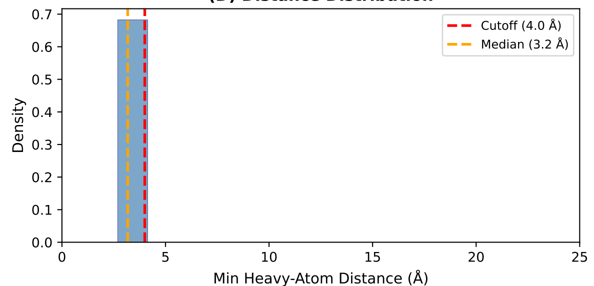
(D) Distance Distribution
