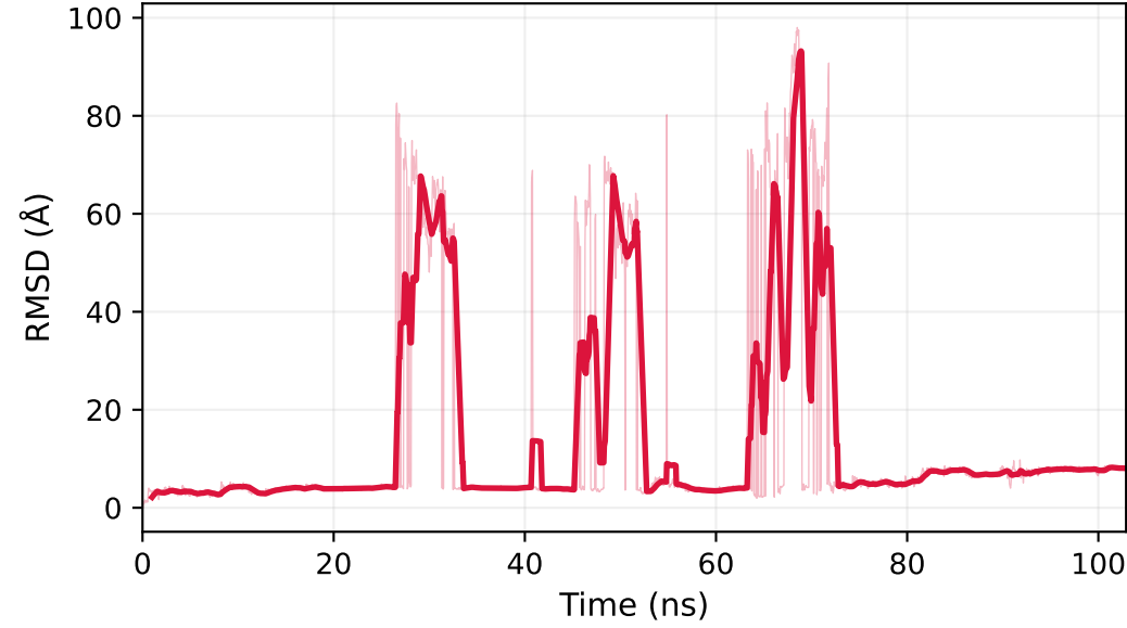
(F) Ligand RMSD
