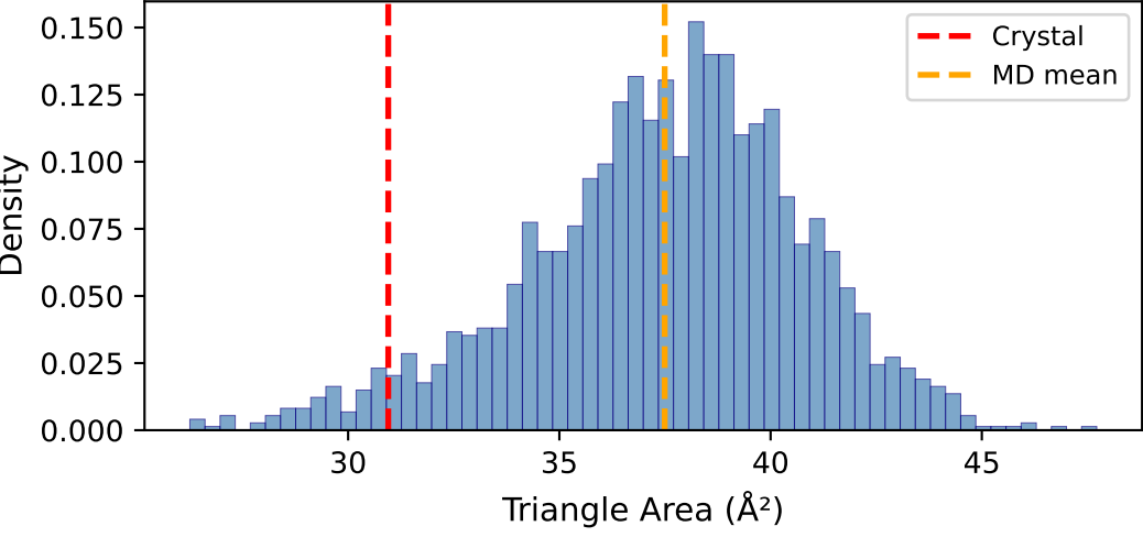
(D) Area Distribution
