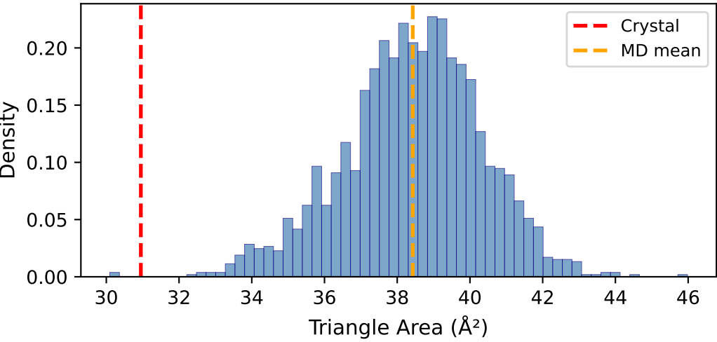
(D) Area Distribution
