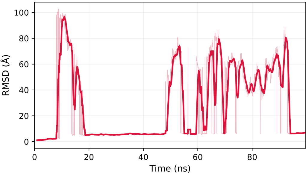
(F) Ligand RMSD
