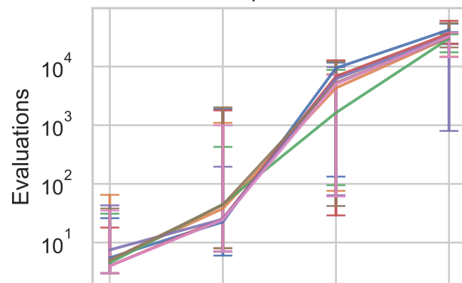
DTrap5/Inverse
