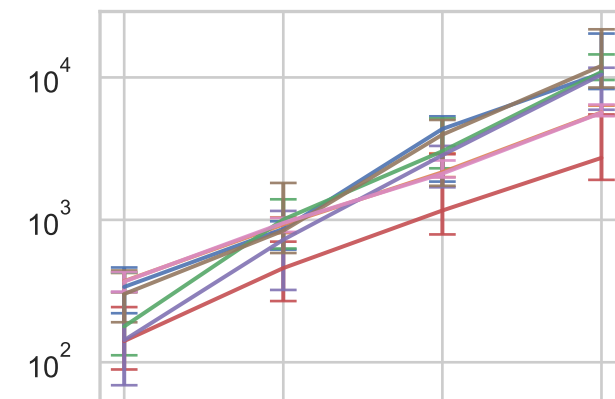
OneMax/ZeroMax
