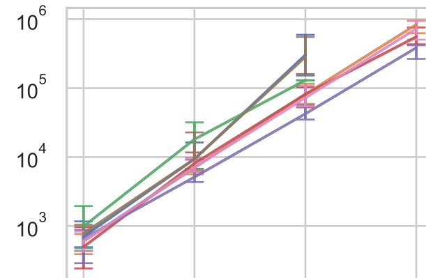
LOTZ
