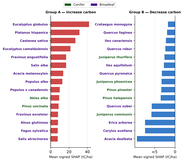
Figura 8.11: Análisis SHAP para el modelo LightGBM entrenado con datos del IFN2 e IFN3 y con variable objetivo c4 (tC/ha) centrándonos en las especies. Se distingue entre conífera o frondosa.
