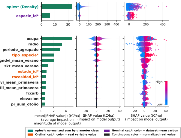
Figura 8.10: Análisis SHAP para el modelo LightGBM entrenado con datos del IFN2 y IFN3 y con variable objetivo c_4 (tC/ha).
