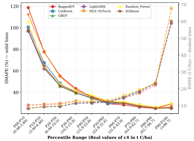
Figura 8.6: Distribución del SMAPE y RMSE en función de la variable objetivo para c4 en deciles.
