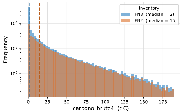
(b) Histograma de la variable carbono_bruto4 en escala logarítmica.
