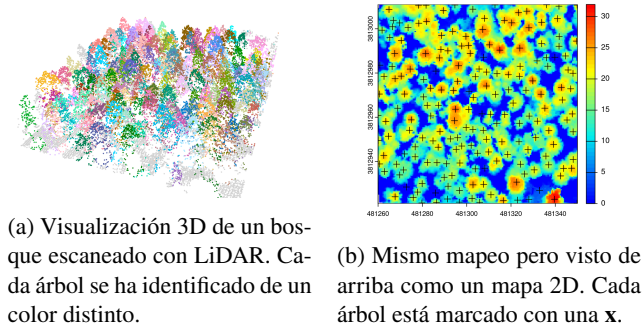
Figura 3.3: Visualización de un bosque escaneado con LiDAR. Vemos las posibilidades de identificar árboles individuales en un entorno forestal denso.
