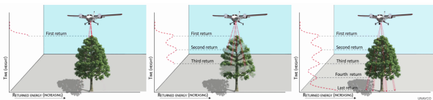
Figura 3.2: Diagrama de el escaneo de un árbol por un sistema LiDAR aerotransportado y los diversos pulsos reflejados. Imagen obtenida de [17].
