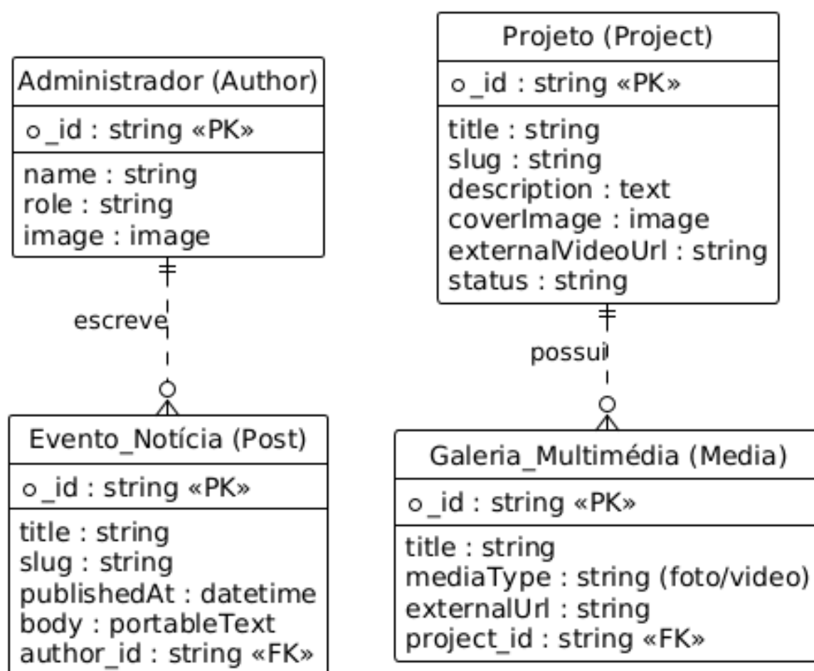
Figura 2 – Diagrama de Coleções e Referências (Sanity CMS)
