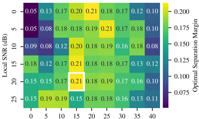
MIT-BIH AF
