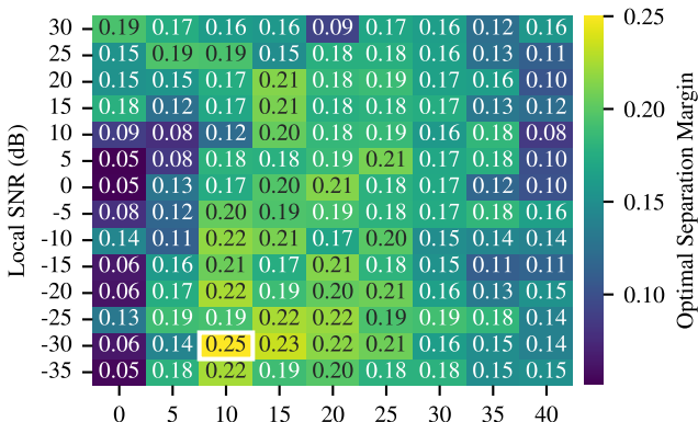
GUdb
