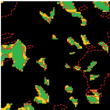
DIS2 errors
