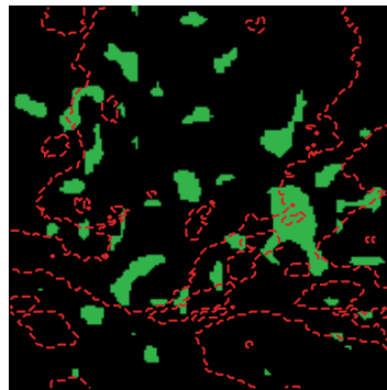
SO baseline
