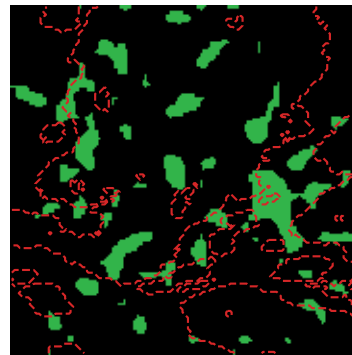
S2 (ours)
