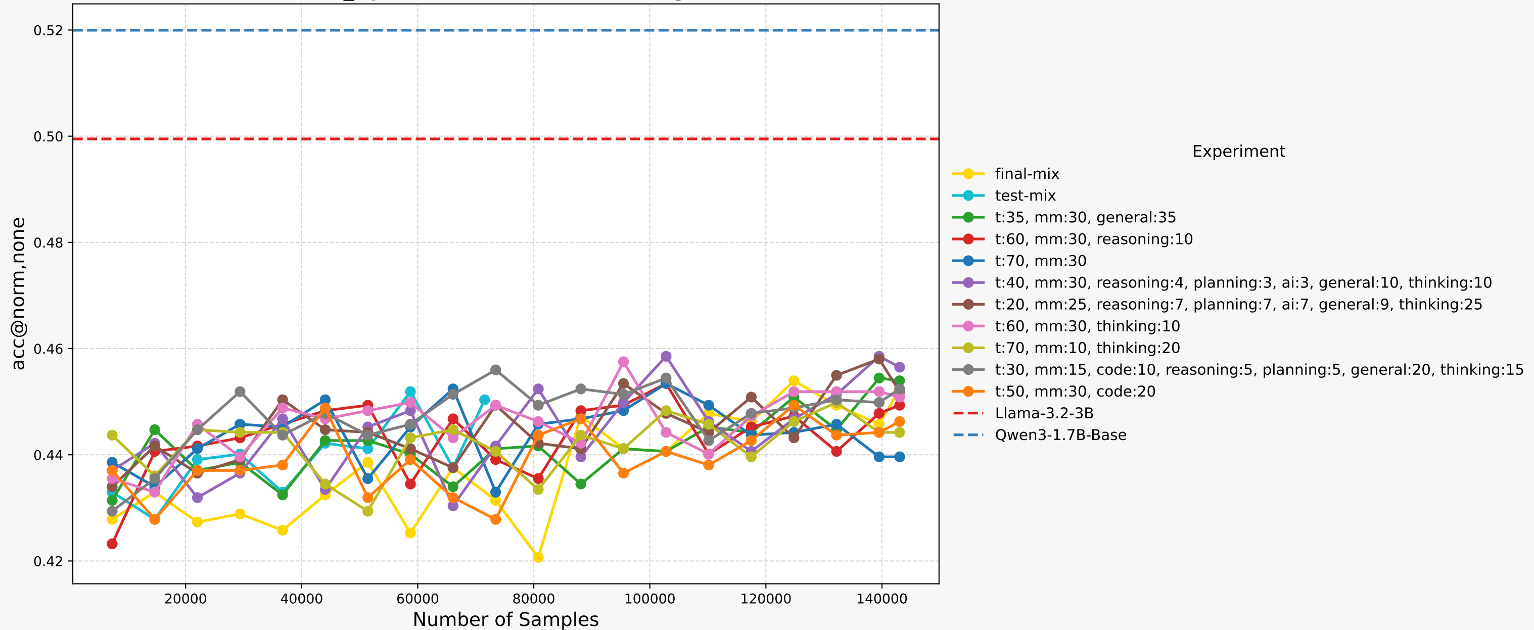
social_iqa Tokenmix Ablation Progress
