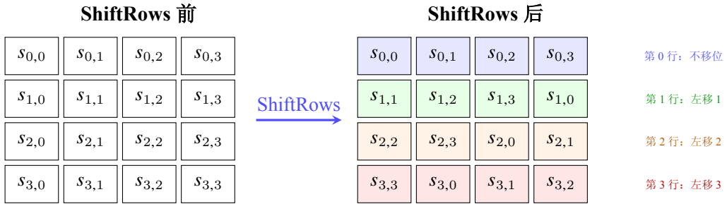
图 2-7 AES ShiftRows 变换示意图。状态矩阵的每一行按行号进行循环左移：第 0 行不移位，第 1 行左移 1 字节，第 2 行左移 2 字节，第 3 行左移 3 字节。不同颜色标注各行移位量
