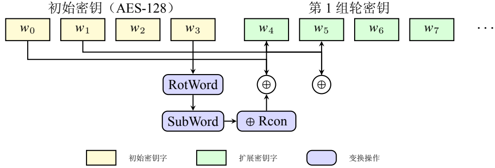
图 2-8 AES-128 密钥扩展流程示意图。初始密钥的 4 个字 w_0-w_3 通过 RotWord、SubWord 和 Rcon 变换递归生成后续字。当 i \bmod 4 = 0 时, w_i = w_{i-4} \oplus \text{SubWord}(\text{RotWord}(w_{i-1})) \oplus \text{Rcon}[i/4] ; 否则 w_i = w_{i-4} \oplus w_{i-1}
