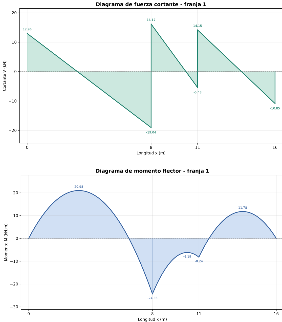
Figura 7: Diagrama de fuerza cortante (DFC, kN) y diagrama de momento flector (DMF, kN.m) de la franja analizada a mano.
