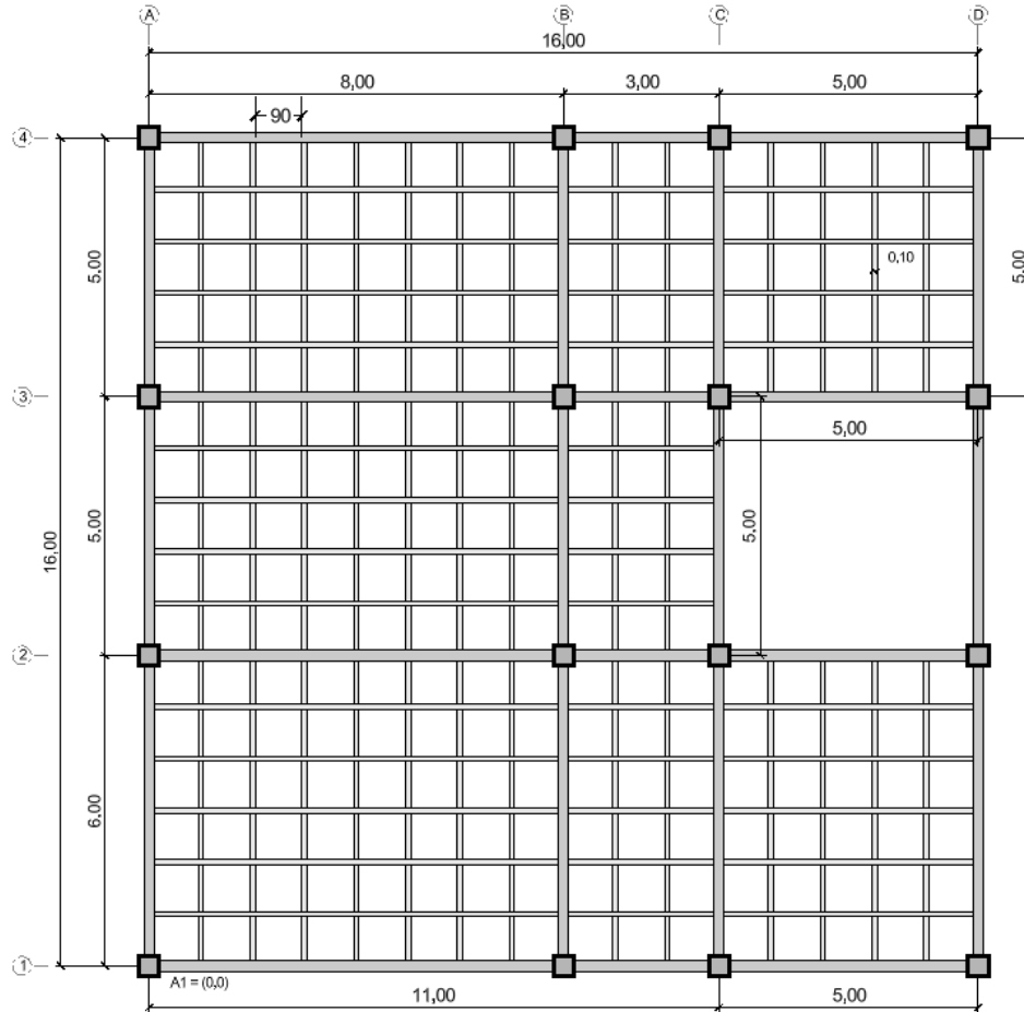
Figura 4: Ubicación en planta de la franja continua analizada, correspondiente a la primera franja horizontal sobre el eje 1 entre A y D.
