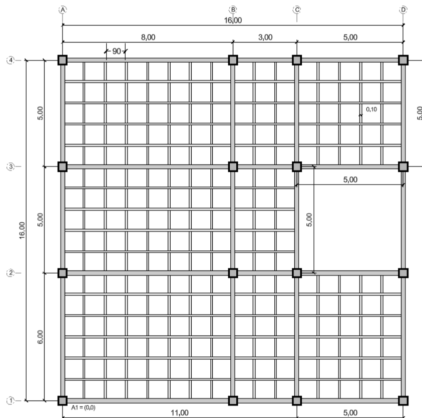
Figura 1: Planta estructural de losa maciza.
