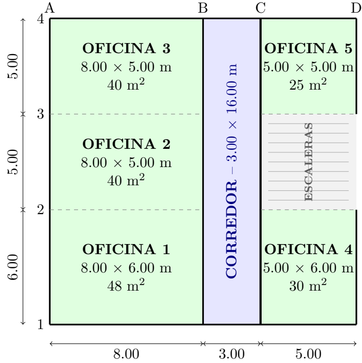
Figura 2: Distribucion arquitectonica en planta.
