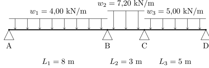
Figura 5: Esquema de la franja continua analizada.
