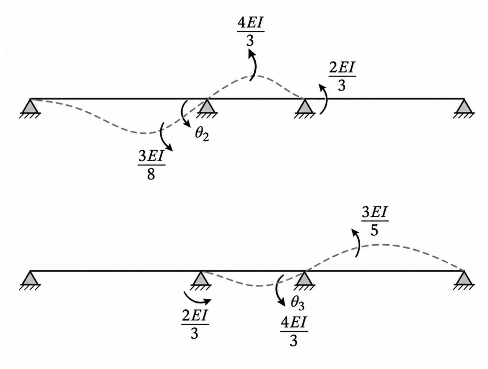
Figura 6: Esquema guía para las ecuaciones de continuidad en los nudos B y C.
