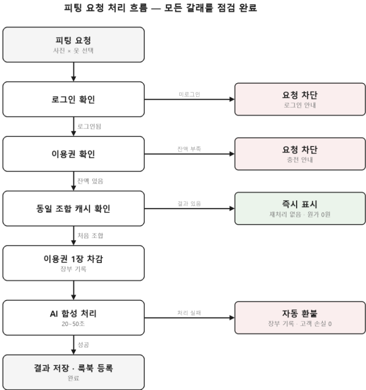
[그림 2] 피팅 요청 처리 흐름 — 점검 완료된 분기 전체
