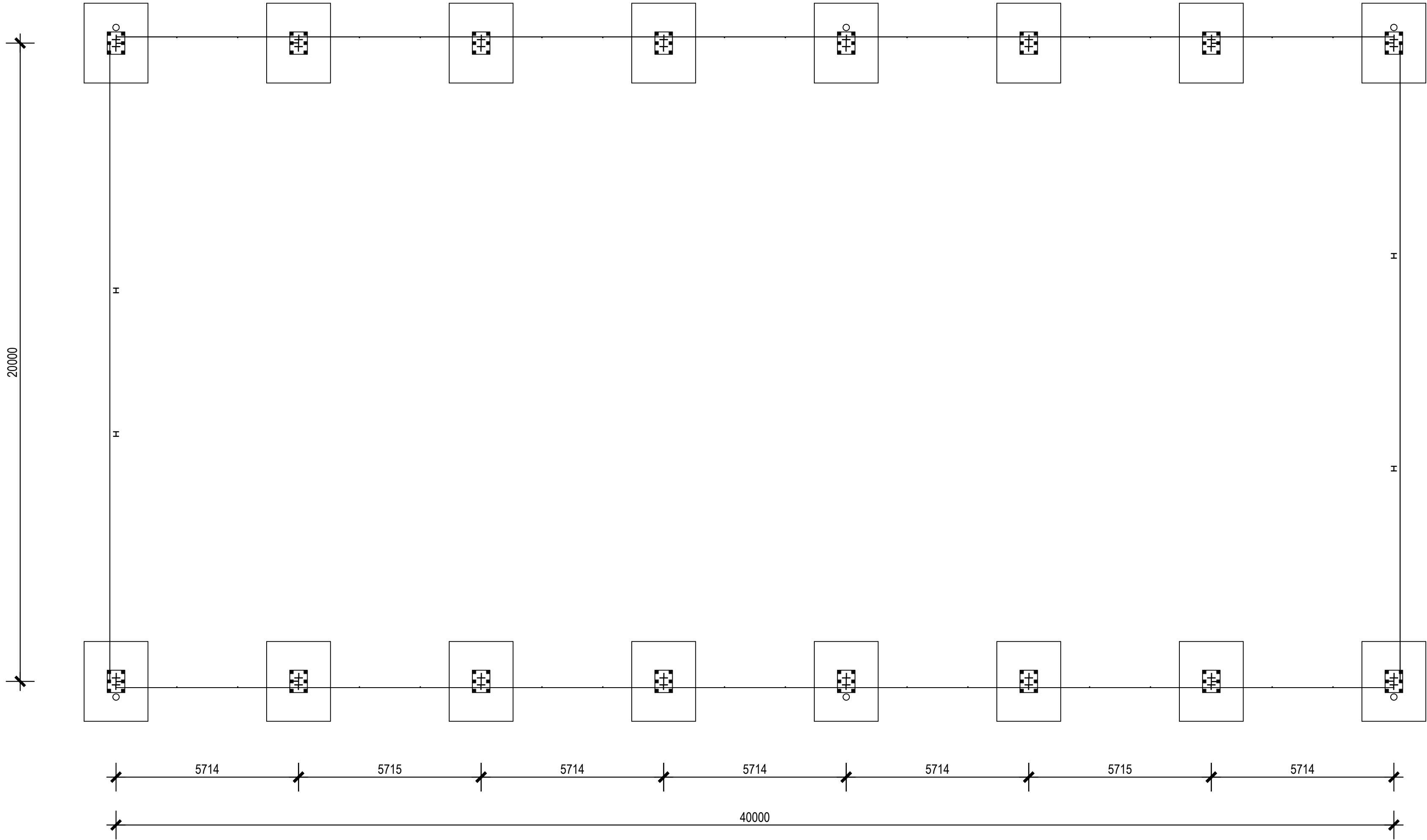
1 PLANTA-BAIXA 1:100
