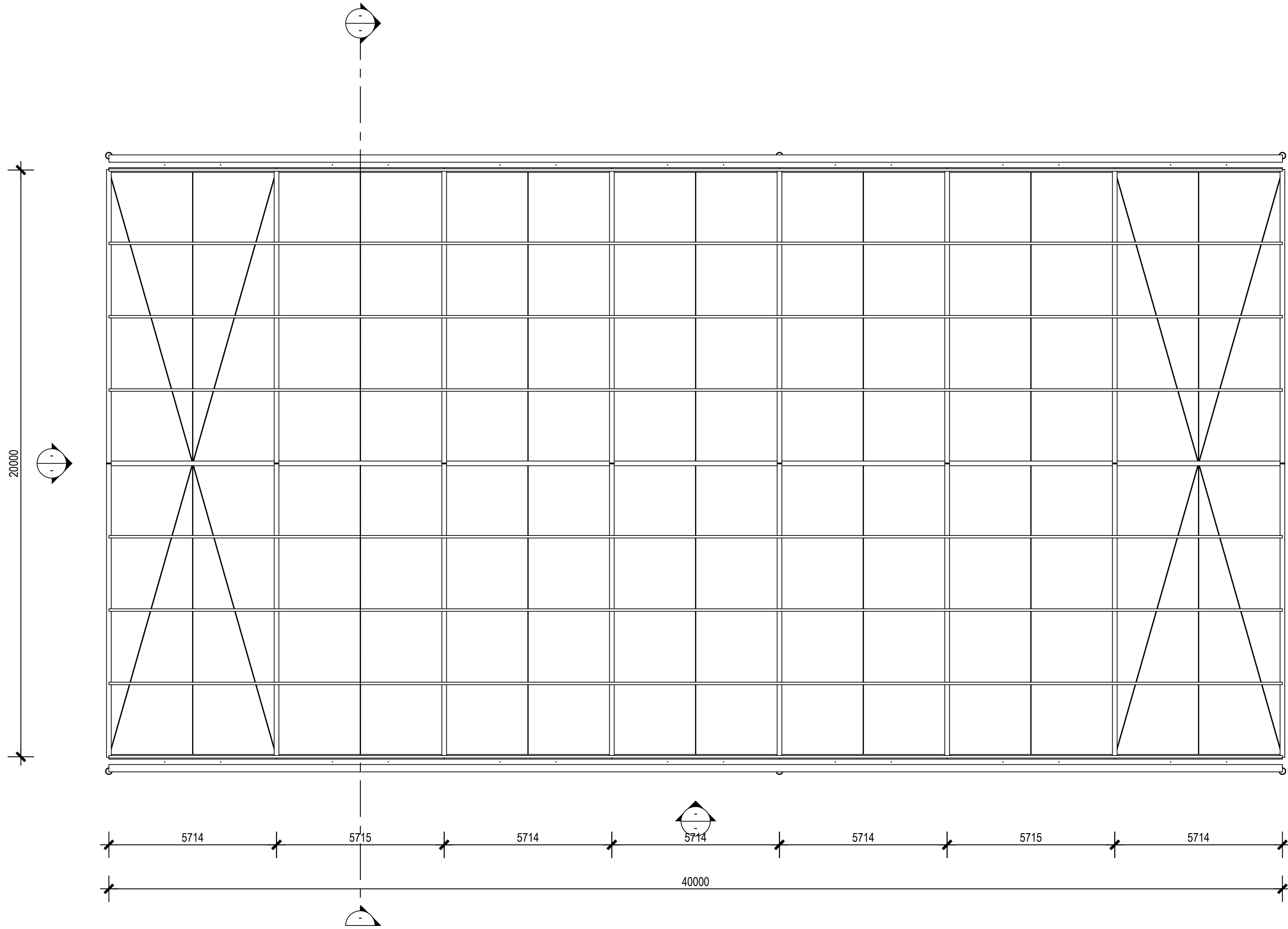
1 PLANTA-COBERTURA 1:100
