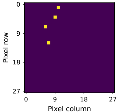
(a) Global MI
