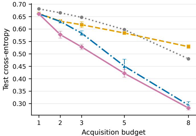
(a) CUBE-NM
