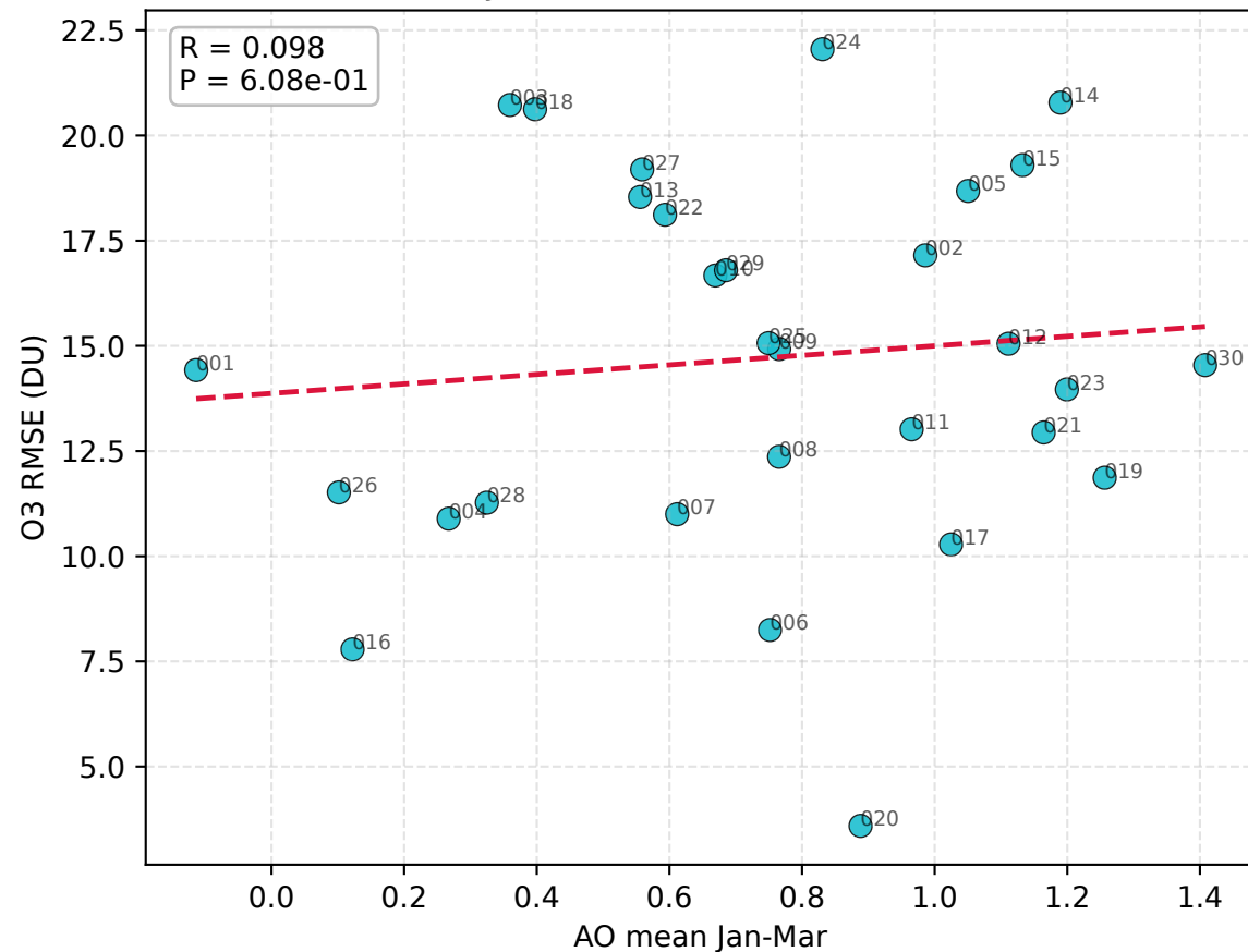
Jan-Mar: AO vs O3 RMSE
