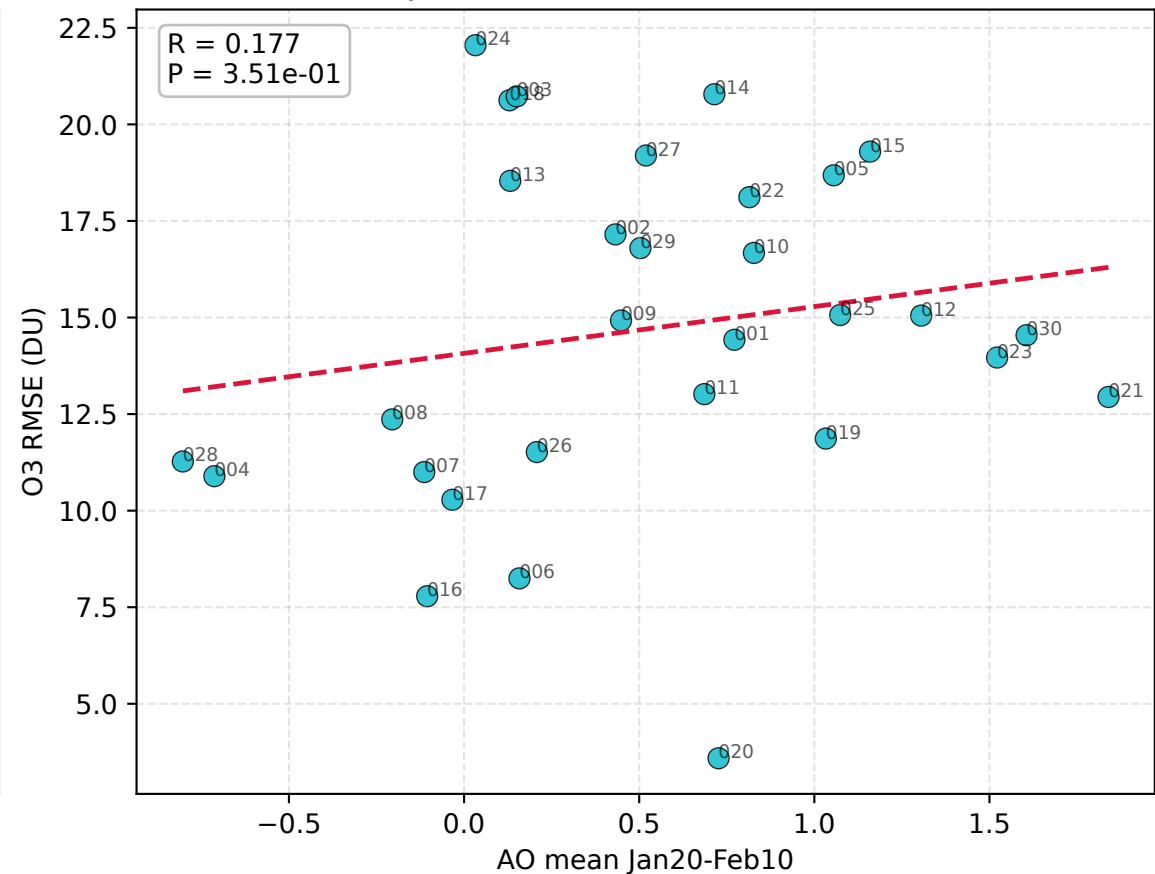
Jan20-Feb10: AO vs O3 RMSE
