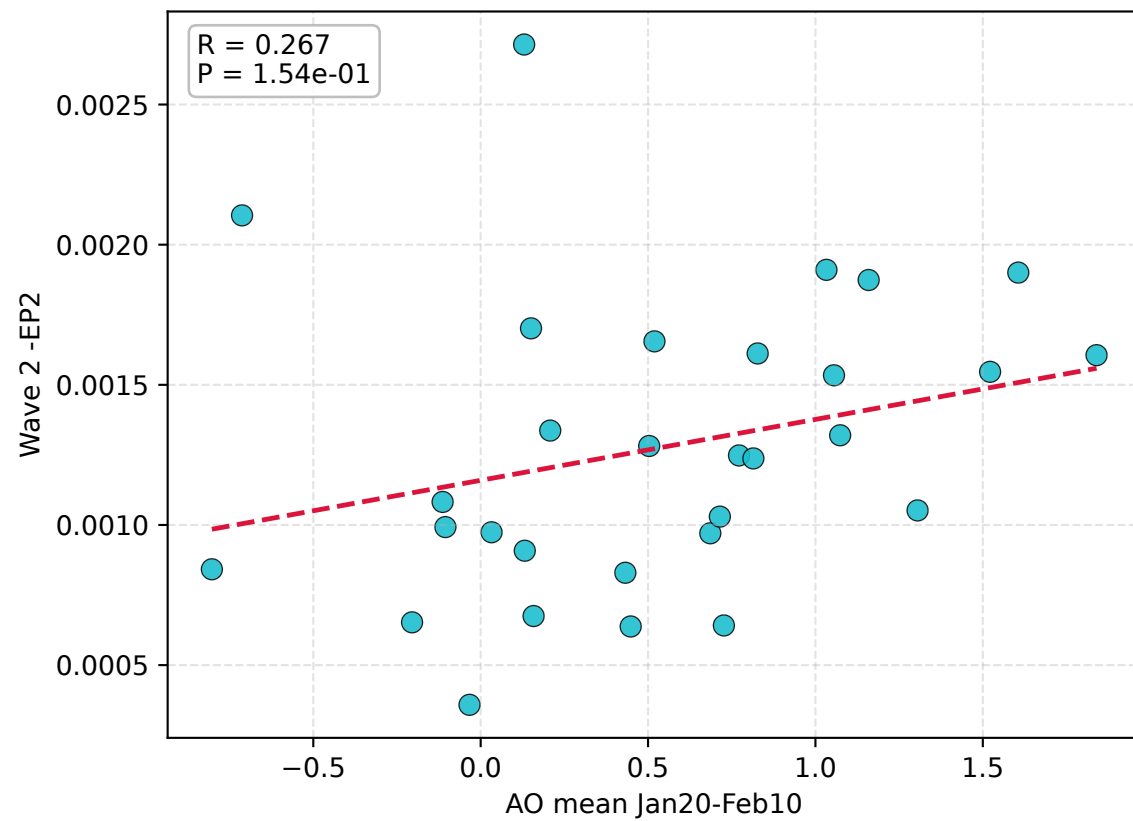
AO vs Wave 2
