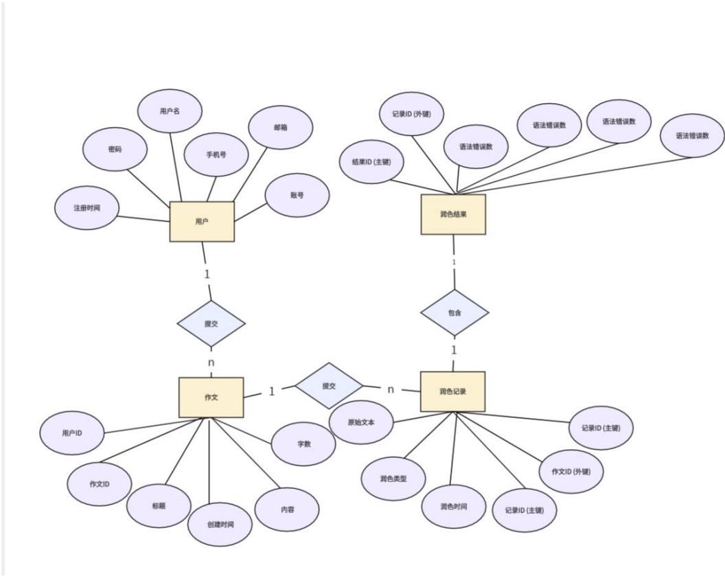
E-R 图
