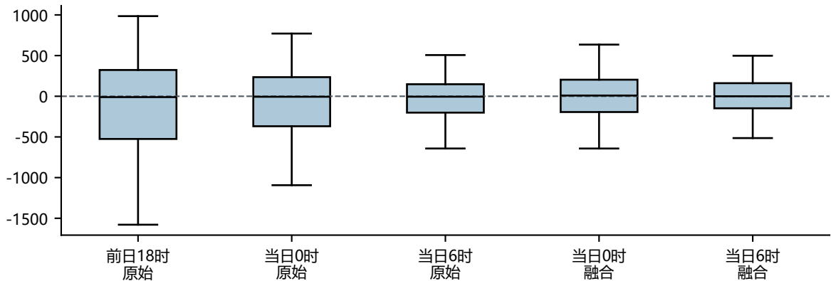
光伏预测误差 / kW
