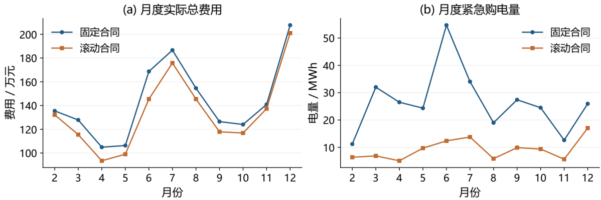
图 6: 波动电价下固定与滚动合同的月度比较
