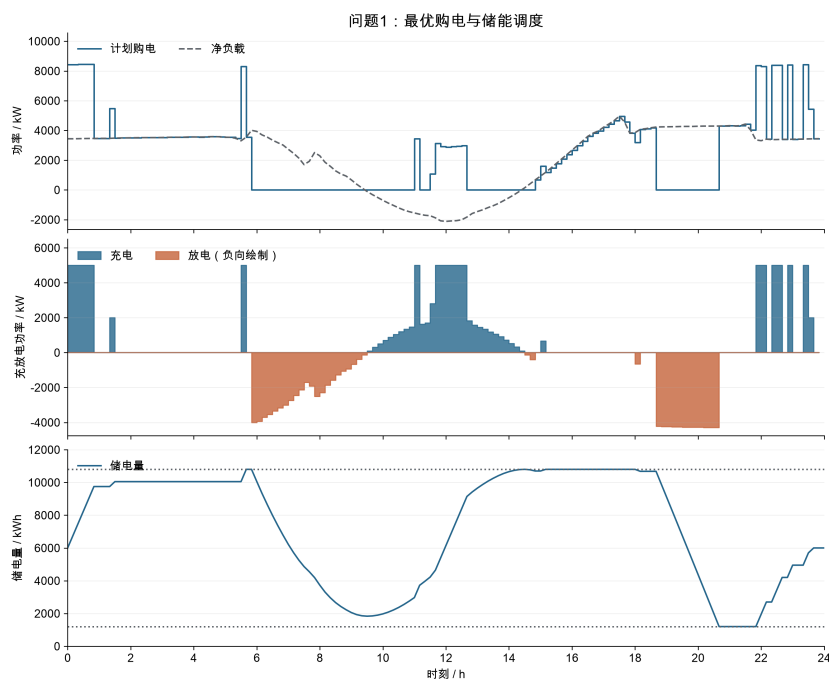
图 2: 代表日购电与储能调度（提供结果）
