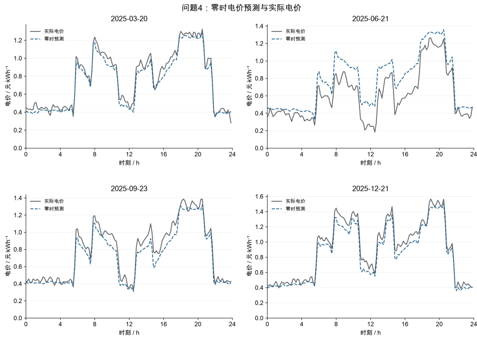
图 5: 指定日期的零时价格预测与实际电价
