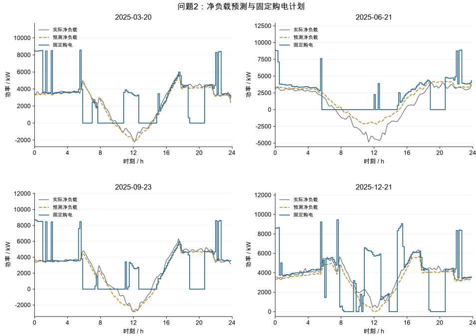
图 3: 指定日期净负载预测与固定购电计划
