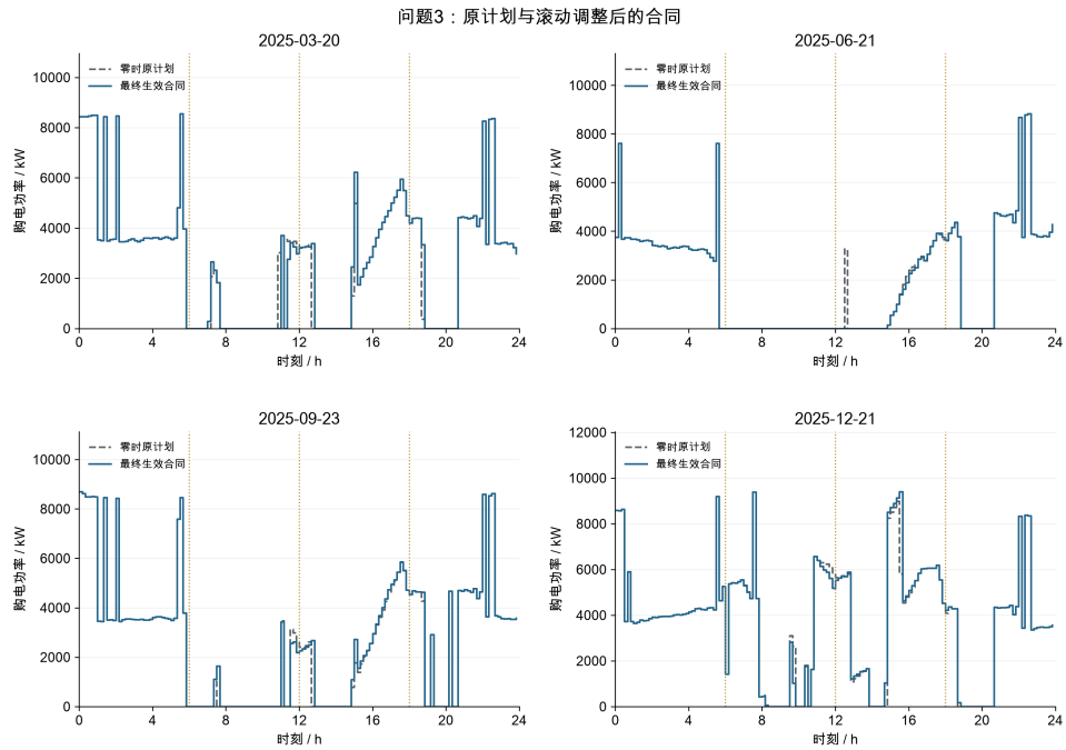
图 4: 指定日期的零时合同与最终调整合同
