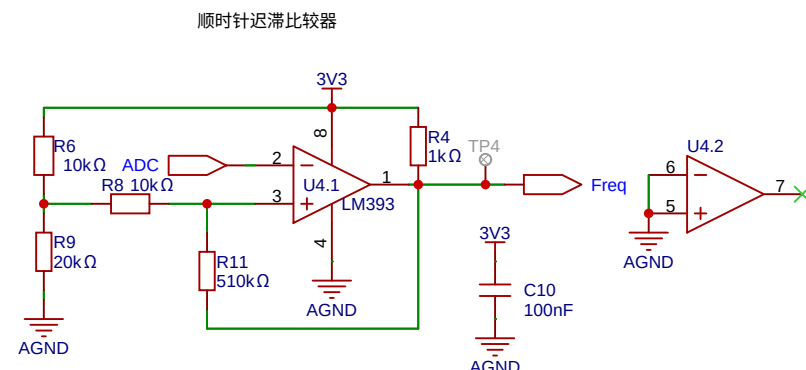
比较器测频电路
