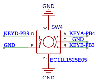
五向开关接口
