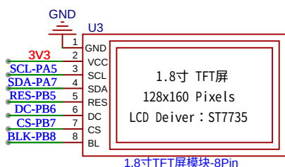
1.8寸TFT屏驱动电路
