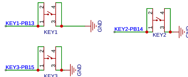
按键控制电路
