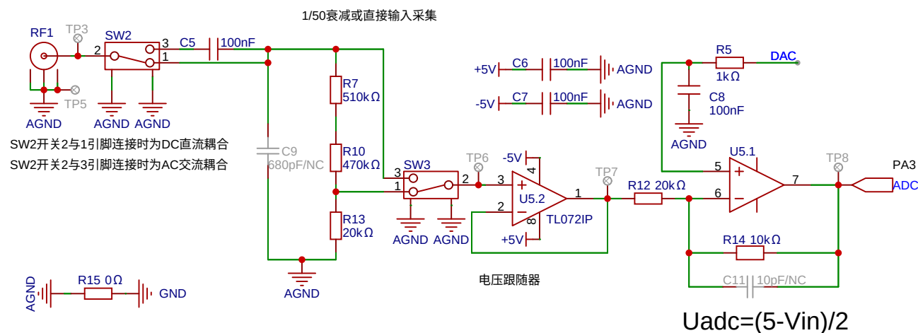
模拟前端处理电路
