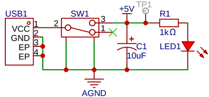
USB电源输入
