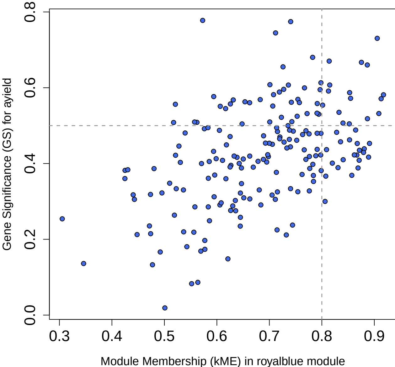
royalblue module cor=0.49, p=3.1e-13
