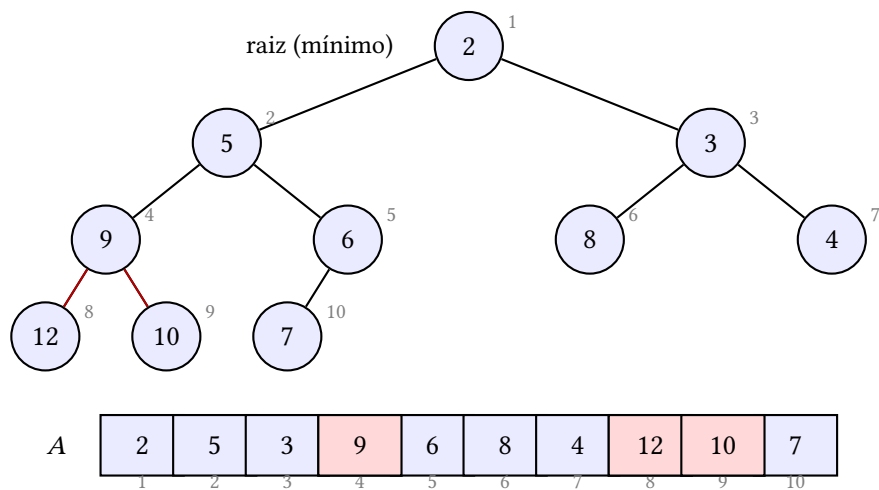
Figura 4.2: Heap com 10 elementos e sua representação em vetor. Para o nó na posição i , o pai está em \lfloor i/2 \rfloor e os filhos em 2i e 2i + 1 . Em destaque, o nó i = 4 e seus filhos 8 e 9.
