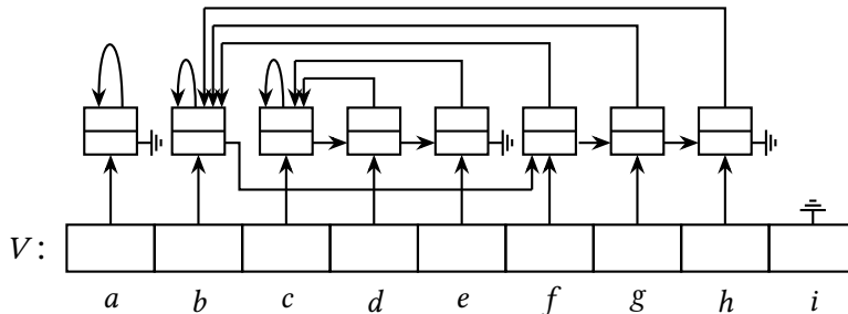
Figura 4.3: Representação com listas ligadas dos subconjuntos \{c, d, e\} , \{a\} e \{b, f, g, h\} do universo \{a, b, c, d, e, f, g, h, i\} .
