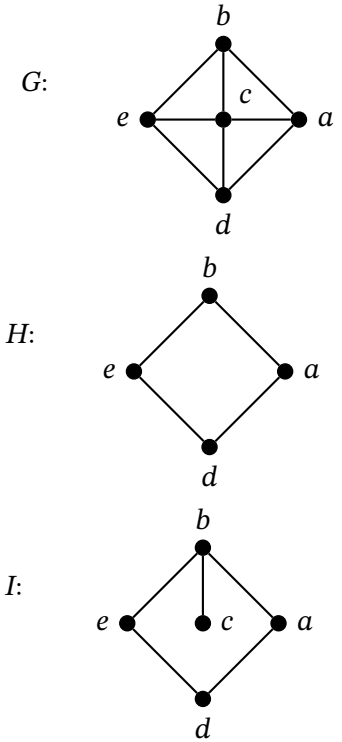
Figura 1.2: diagrama dos grafos G , H e I .
