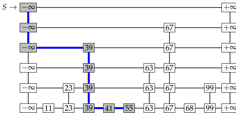
Figura 4.2: o caminho da busca por 55 na skip list da Figura 4.1.
