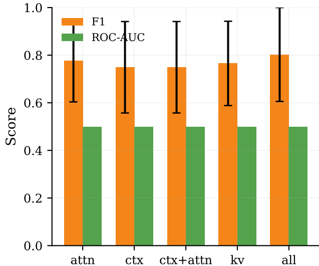
Context-Bucket-Held-Out
