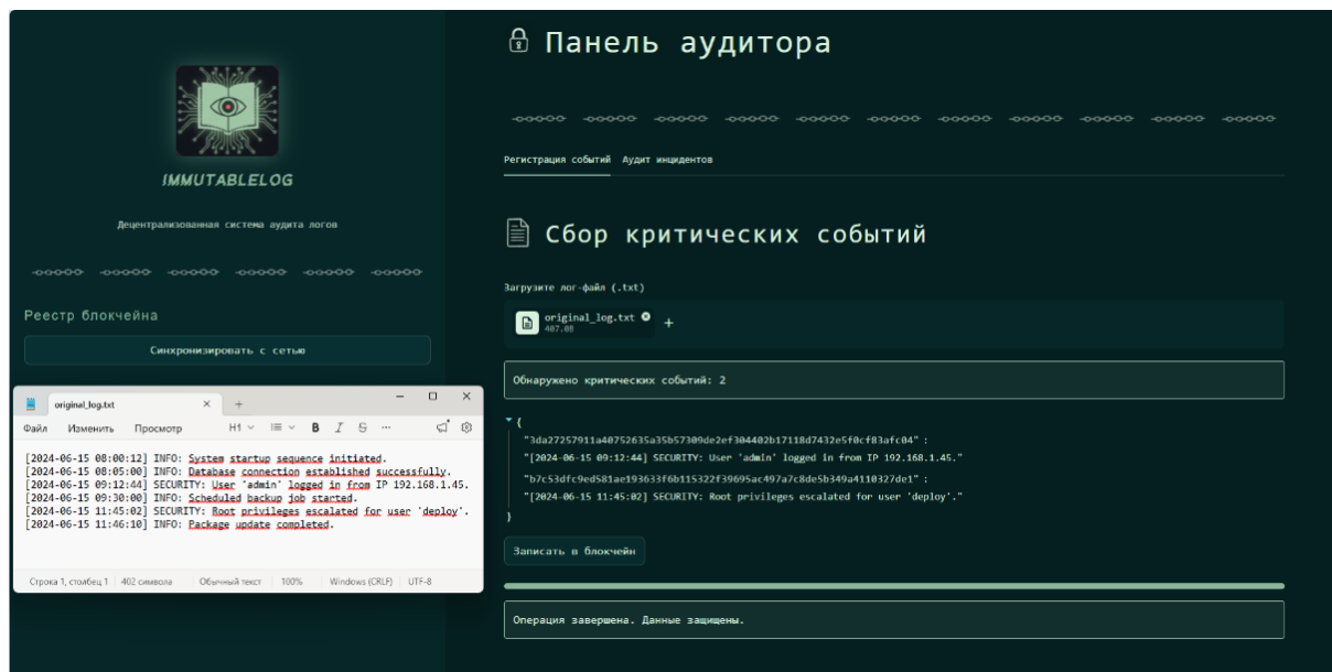
Рисунок 2 – Регистрация событий: две записи категории SECURITY, отображение хэшей и исходных строк, индикация завершения записи в блокчейн
