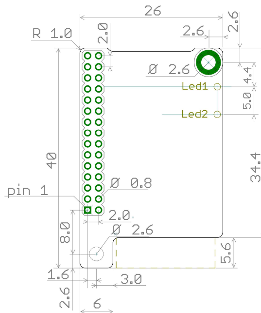
ESP32-MEZZA25-R ESP32-MEZZAR
