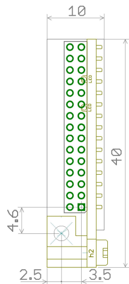
ESP32-MEZZA25-VR3 ESP32-MEZZA25-13
