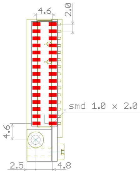
ESP32-MEZZA25-VR4-SMD ESP32-MEZZA25-14S
