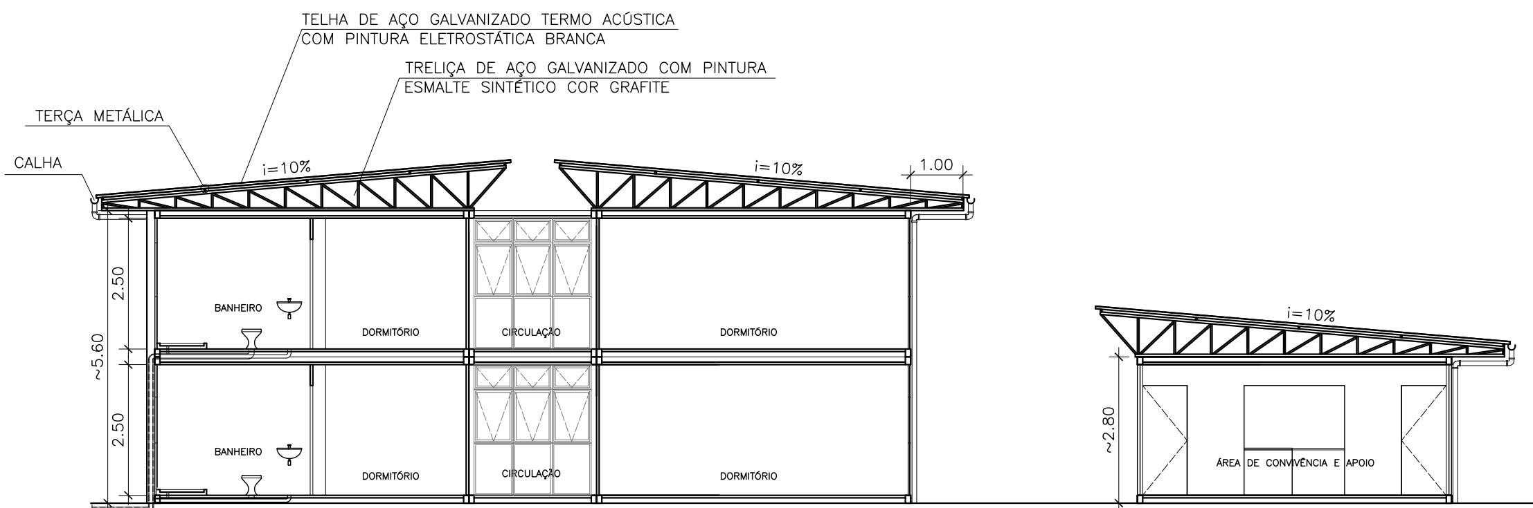
4 CORTE TRANSVERSAL AA ESC.: 1:100
