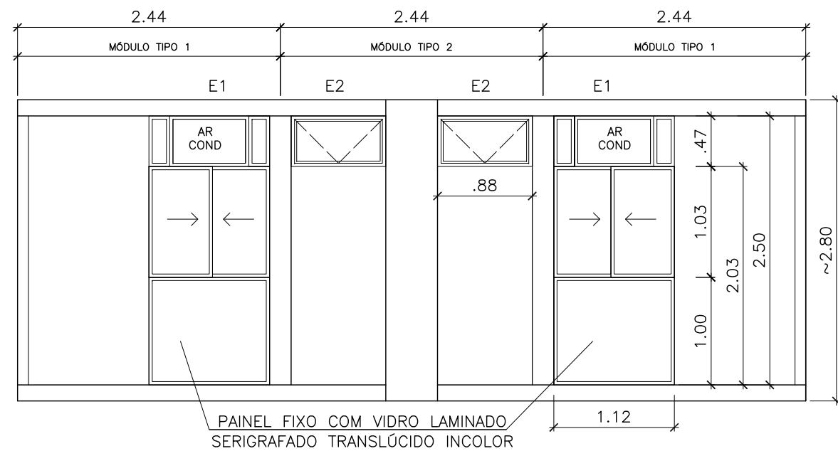
7 ELEVÇÃO TIPO DOS MÓDULOS DE ALOJAMENTO ESC.: 1:50
