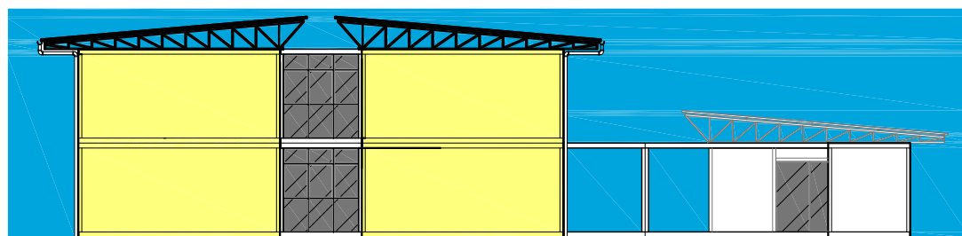
3 ALOJAMENTO – FACHADA NORDESTE ESC.: 1:200
