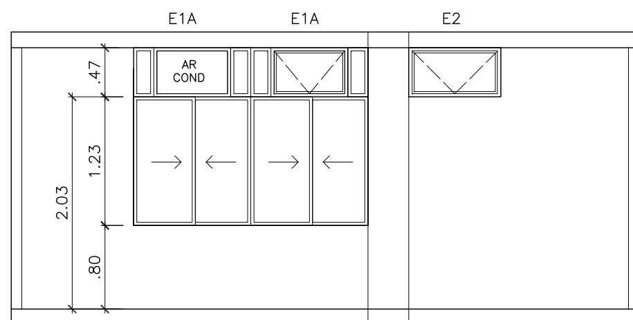
8 ELEVÇÃO TIPO MÓDULOS DE ALOJAMENTO PNE ESC.: 1:50
