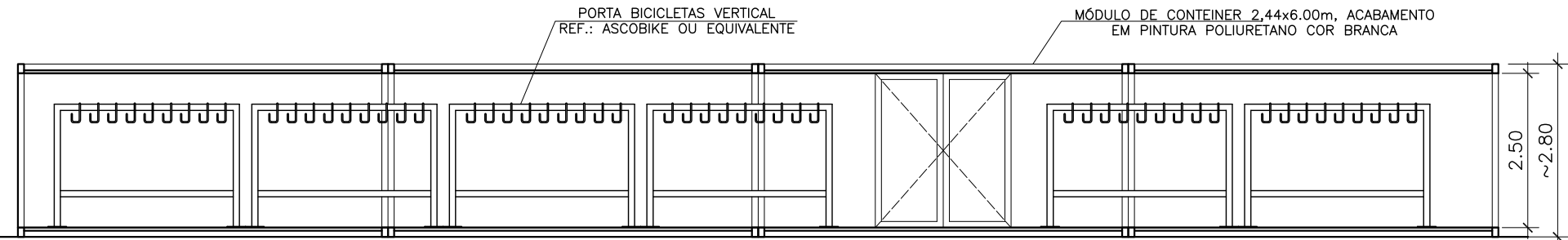
6 CORTE CC – BICICLETÁRIO ESC.: 1:100
