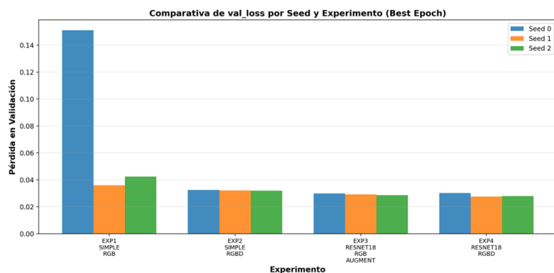
Ilustración 5-6. Comparativa de val_loss por ejecución (seed) y experimento, evaluado en best_epoch (seleccionado por máximo val_success).
