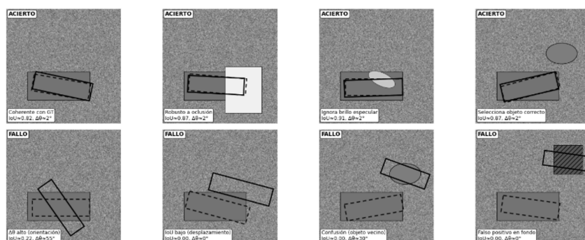
Ilustración 4-5. Galería cualitativa: 4 aciertos + 4 fallos con explicación del tipo de fallo. Panel 2x4 con superposición de rectángulos de agarre: GT (línea discontinua) y Pred (línea continua). En los aciertos se observa alto solape y baja discrepancia angular; en los fallos se ilustran patrones típicos: \Delta\theta elevado (orientación incorrecta), IoU bajo (desplazamiento/escala), confusión de instancia (agarre en objeto vecino) y falso positivo sobre fondo. Se muestran valores aproximados de IoU y \Delta\theta como guía interpretativa. (Elaboración propia).
