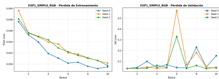
Ilustración 5-1. Curvas de pérdida ( train_loss y val_loss ) para EXP1 (SimpleGraspCNN, RGB).
