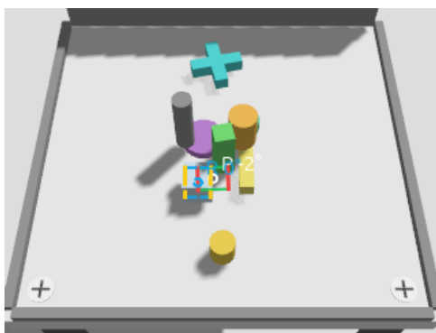
Ilustración 5-17. Resultado de inferencia del modelo EXP3_RESNET18_RGB_AUGMENT sobre la imagen simulada, mostrando la hipótesis de agarre estimada y su representación visual en el panel de integración.
