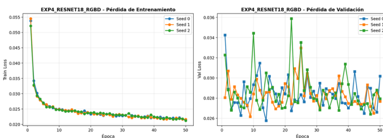
Ilustración 5-4. Curvas de pérdida ( train_loss y val_loss ) para EXP4 (ResNet18Grasp, RGB-D).
