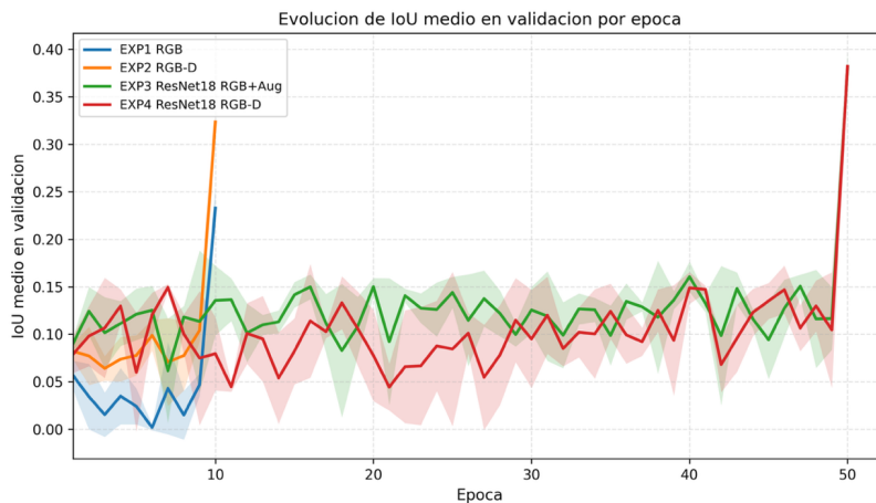
Ilustración 5-8. Evolución del IoU medio en validación por época para las cuatro configuraciones experimentales.
