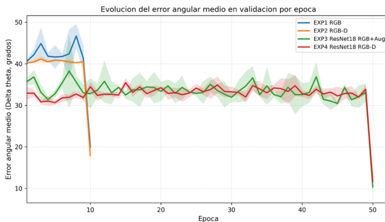
Ilustración 5-9. Evolución del error angular medio ( \Delta\theta , en grados) en validación por época para las cuatro configuraciones experimentales.
