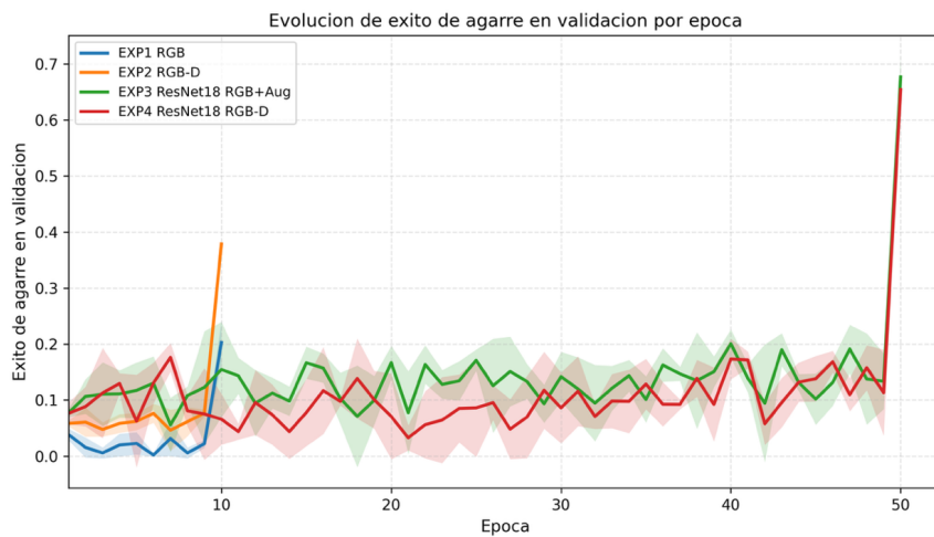
Ilustración 5-7. Evolución del éxito de agarre en validación (val_success) por época para las cuatro configuraciones experimentales.
