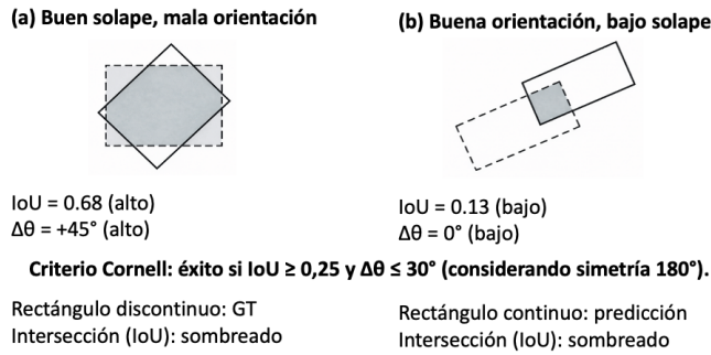
Ilustración 3-6. Interpretación geométrica de IoU y \Delta\theta en rectángulos orientados. En ambos paneles se compara el rectángulo de referencia (ground truth, GT, línea discontinua) frente al rectángulo predicho (predicción, línea continua). El área sombreada representa la intersección usada para el cálculo de IoU. (a) Ejemplo con IoU alto, pero \Delta\theta alto (buen solape, mala orientación). (b) Ejemplo con IoU bajo, pero \Delta\theta bajo (buena orientación, bajo solape por desplazamiento). (Elaboración propia).
