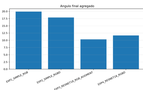
Ilustración 5-12. Error angular medio final ( \Delta\theta en grados) en validación, agregado por experimento ( media ± desviación estándar sobre semillas), bajo el criterio de best_epoch .
