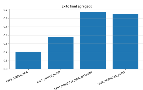
Ilustración 5-10. Éxito final de agarre en validación ( val_success ), agregado por experimento ( media ± desviación estándar sobre semillas), seleccionando en cada ejecución best_epoch por máximo val_success .
