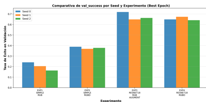
Ilustración 5-5. Comparativa de val_success por ejecución ( seed ) y experimento, tomando el valor en la mejor época ( best_epoch ) seleccionada por máximo val_success .
