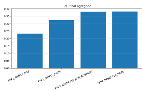
Ilustración 5-11. IoU medio final en validación, agregado por experimento ( media ± desviación estándar sobre semillas) bajo el criterio de selección de best_epoch .
