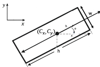
Ilustración 3-5. Parámetros del rectángulo de agarre (C_x, C_y, w, h, \theta) sobre una imagen. El agarre se representa como un rectángulo orientado en el plano imagen: (C_x, C_y) denota el centro en píxeles, w la dimensión perpendicular al eje principal (apertura efectiva en imagen), h la dimensión a lo largo del eje principal (longitud útil de contacto) y \theta el ángulo de orientación del eje principal (asociado a h ) respecto al eje x de la imagen. (Elaboración propia, basada en Platt, 2023)
