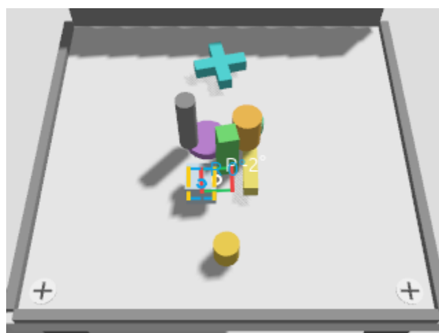
Ilustración 5-17. Resultado de inferencia del modelo EXP3_RESNET18_RGB_AUGMENT sobre la imagen simulada, mostrando la hipótesis de agarre estimada y su representación visual en el panel de integración.
