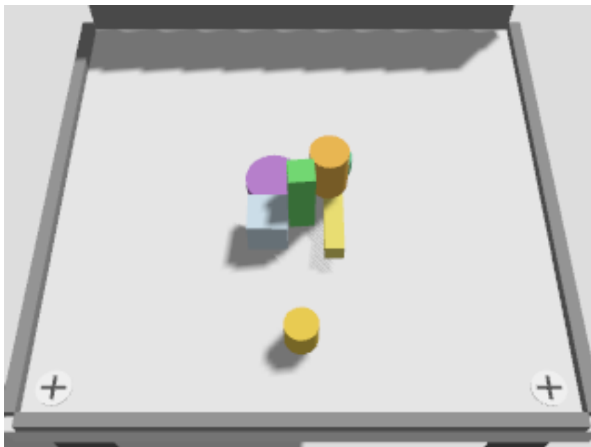
Ilustración 5-16. Evidencia funcional del pipeline percepción–publicación–consumo en ROS 2, donde la hipótesis de agarre generada por el detector se transforma en una pose ejecutable y es procesada por el subsistema de planificación a través de la interfaz definida para la integración con MoveIt.
