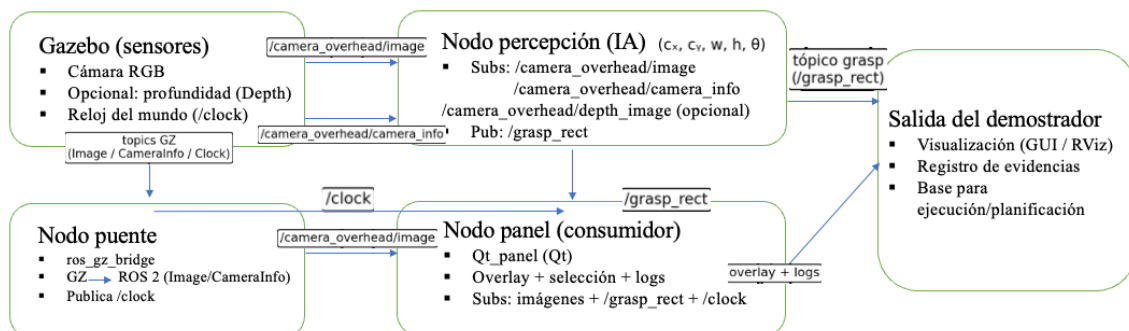
Ilustración 4-6. Arquitectura ROS 2 del entorno simulado (nodos y tópicos).
