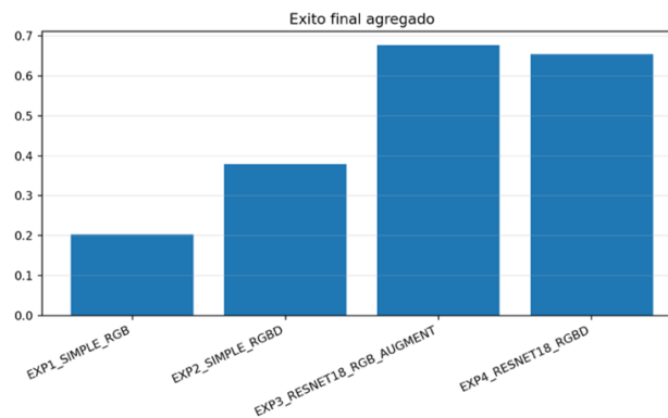
Ilustración 5-10. Éxito final de agarre en validación ( val_success ), agregado por experimento (media \pm desviación estándar sobre semillas), seleccionando en cada ejecución best_epoch por máximo val_success .
