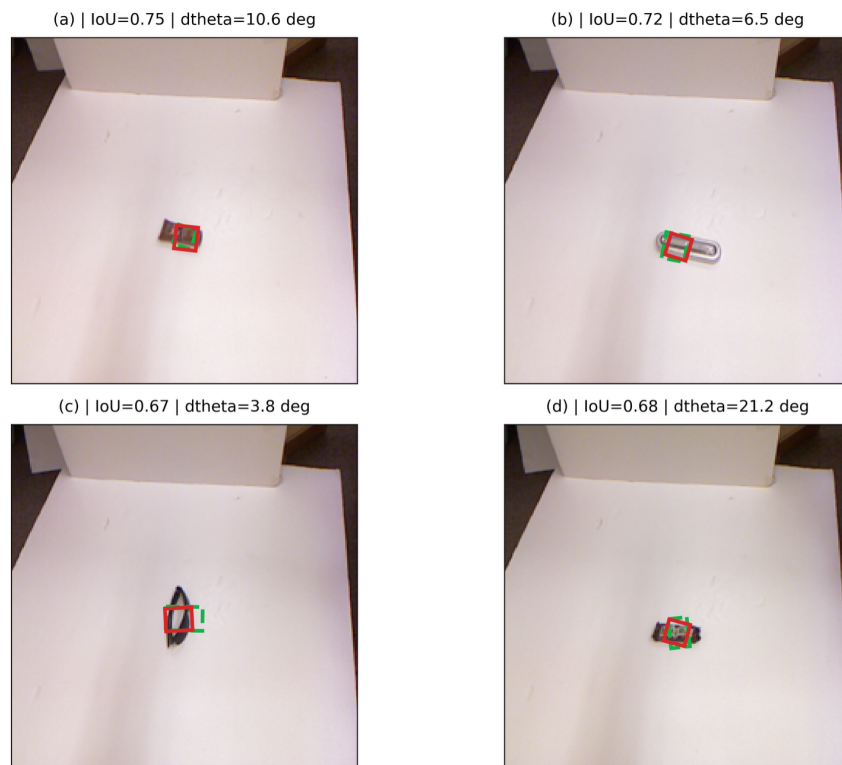
Ilustración 5-13. Aciertos representativos en validación para el modelo EXP3_RESNET18_RGB_AUGMENT (seed 0), con superposición entre el GT seleccionado (verde discontinuo) y la predicción (rojo continuo).
