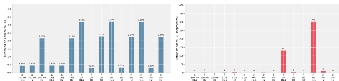
Figura 9. Análise de tráfego PCAP: overhead de protocolo e contagem de retransmissões.
