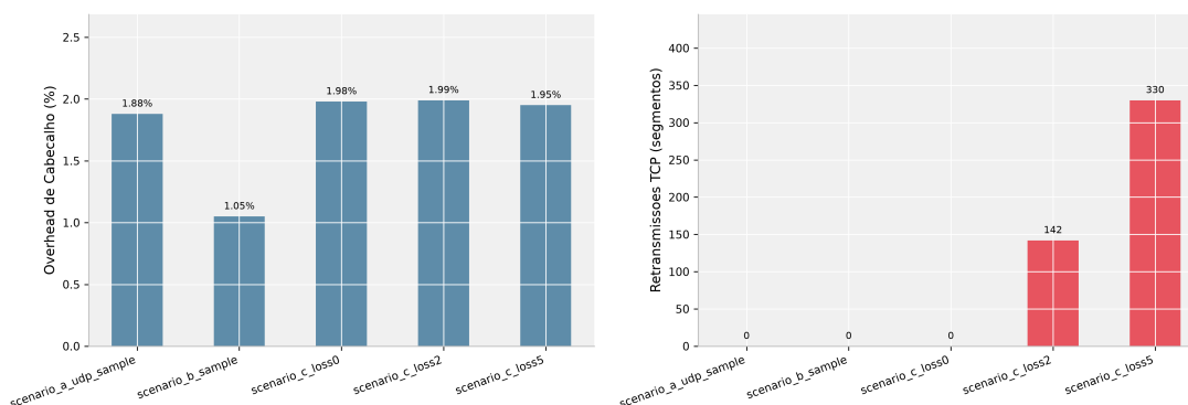
Figura 9. Análise de tráfego PCAP: overhead de protocolo e contagem de retransmissões.
