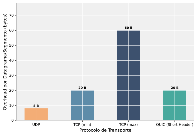
Figura 4. Comparação do overhead de cabeçalho de transporte entre UDP, TCP e QUIC.
