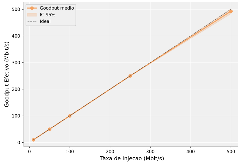
Figura 2. Vazão efetiva do UDP puro em função da taxa de injeção.
