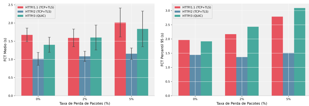
Figura 7. FCT médio e percentil p95 sob perdas de pacotes de 0%, 2% e 5%.
