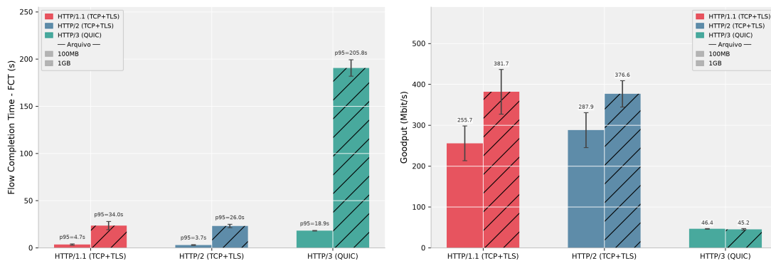
Figura 5. FCT e goodput para transferências de 100 MB e 1 GB em canal estável.
