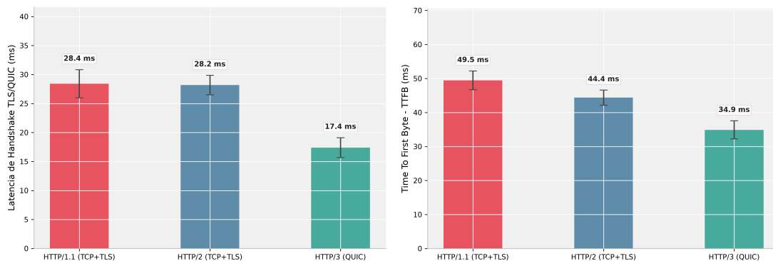
Figura 6. Comparação de latência de handshake e TTFB no Cenário B.
