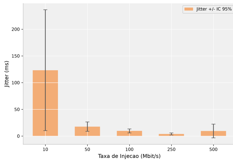
Figura 3. Jitter do UDP puro em função da taxa de injeção.
