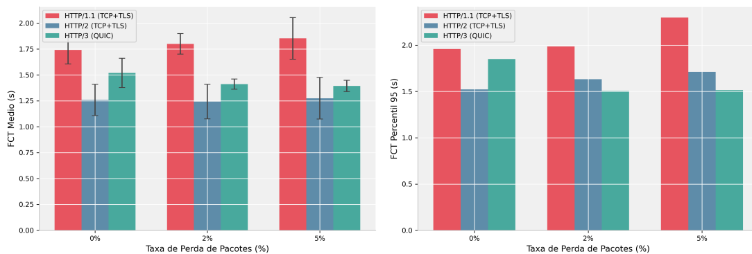
Figura 7. FCT médio e percentil p95 sob perdas de pacotes de 0%, 2% e 5%.
