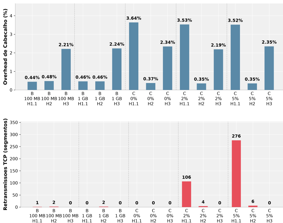
Figura 9. Análise de tráfego PCAP: overhead de protocolo (superior) e contagem de retransmissões TCP (inferior).
