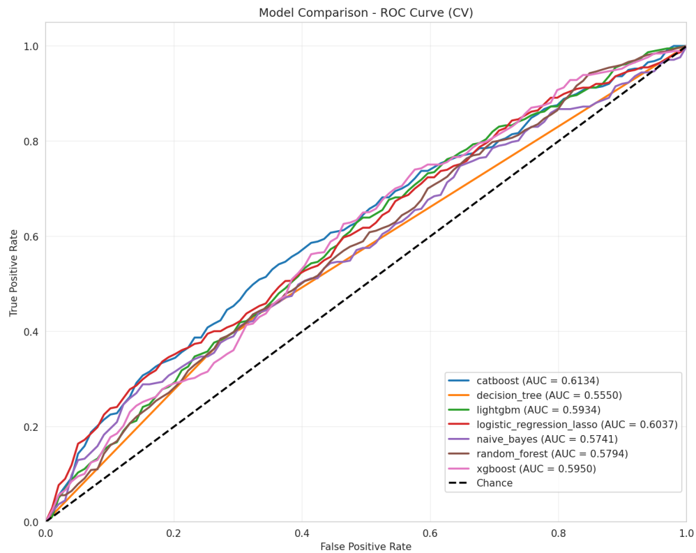
Figura 39: Comparación de curvas ROC - Experimento 3
