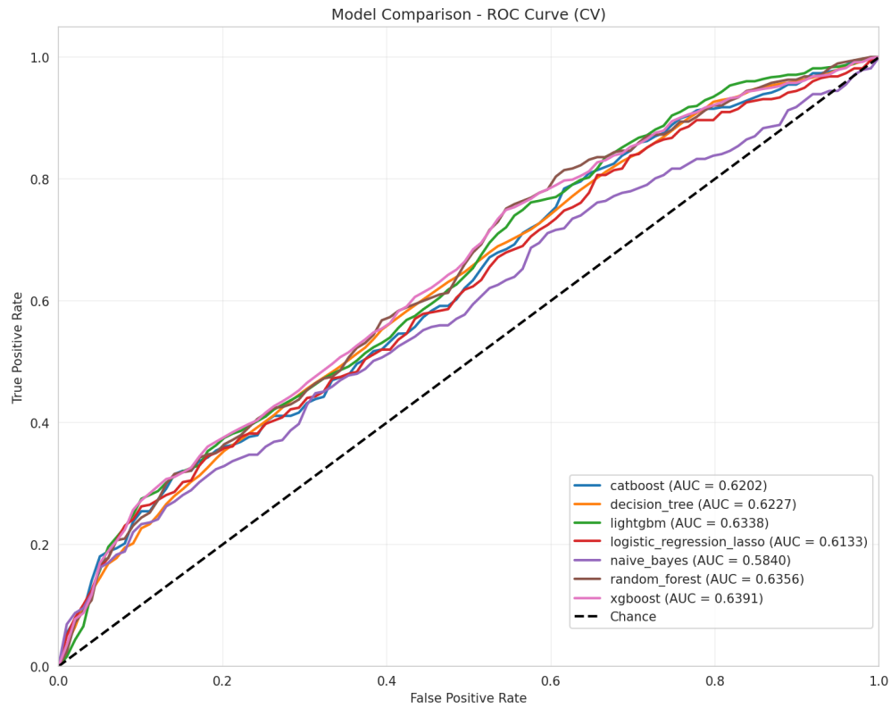
Figura 41: Comparación de curvas ROC - Experimento 5 (Modelo Campeón)
