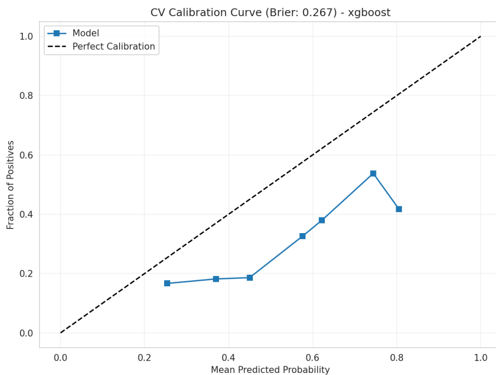
Figura 43: Curva de calibración - Modelo Campeón
