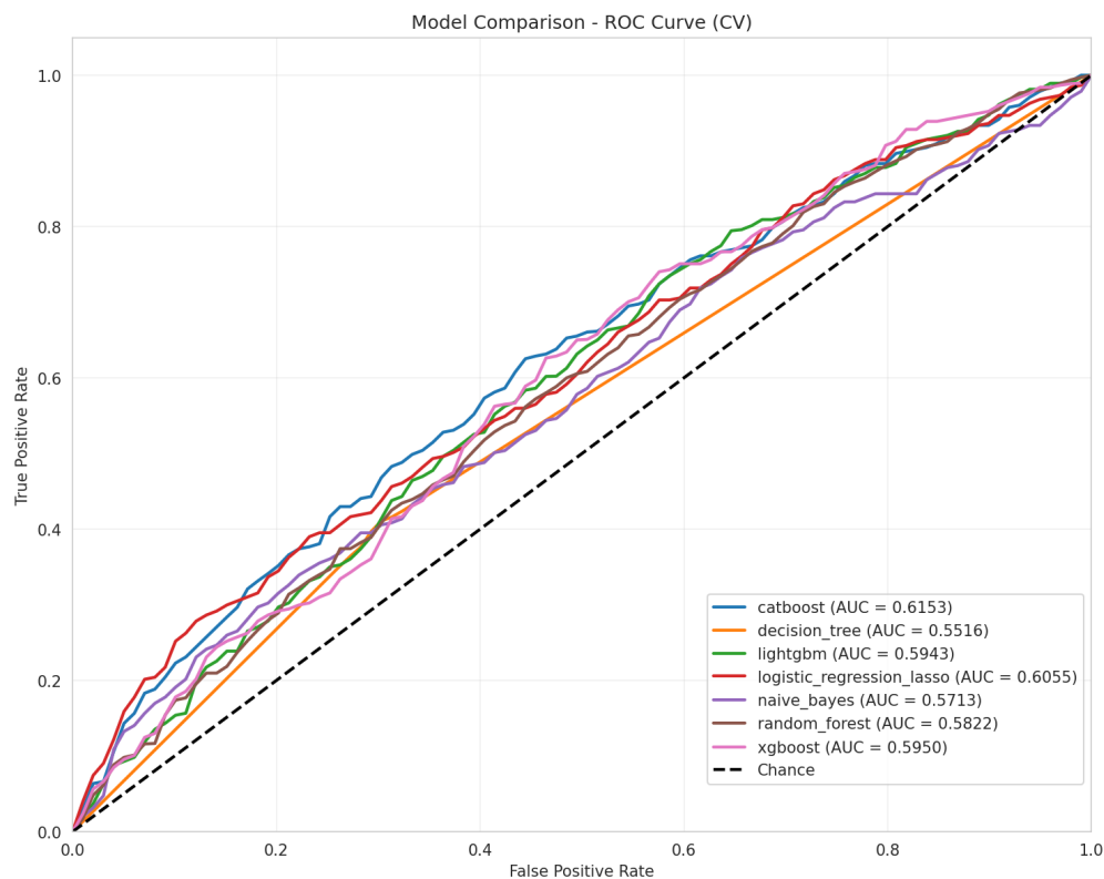
Figura 37: Comparación de curvas ROC - Experimento 1
