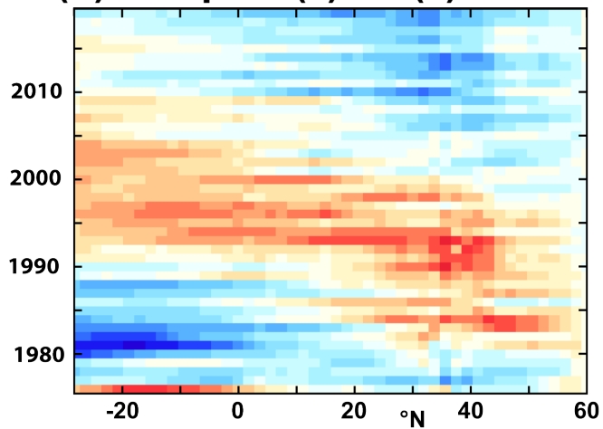
(d) GS1p0 \Psi(z) - \langle \Psi(z) \rangle
