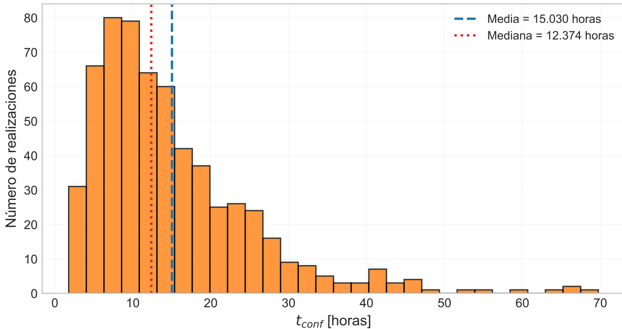
Distribución de t_{conf} (T = 0,1 K, N = 600)
